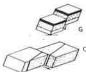
Fallas: G: De Gravedad (directa) D: de Desgarre
