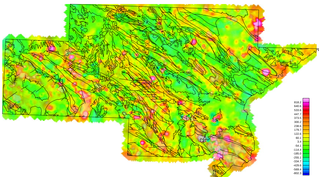
Figura 6-344. Mapa aditivo de Pb-Zn-Cu. Escala log-lineal
