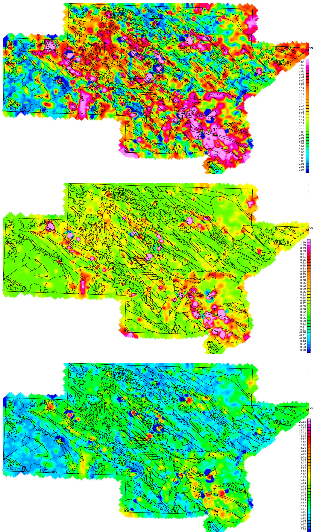
Figura 6-260. Mapas de distribución de Cd con escala ecualizada a partir del histograma, con escala de distribución normal y con escala log-lineal (de arriba abajo)
