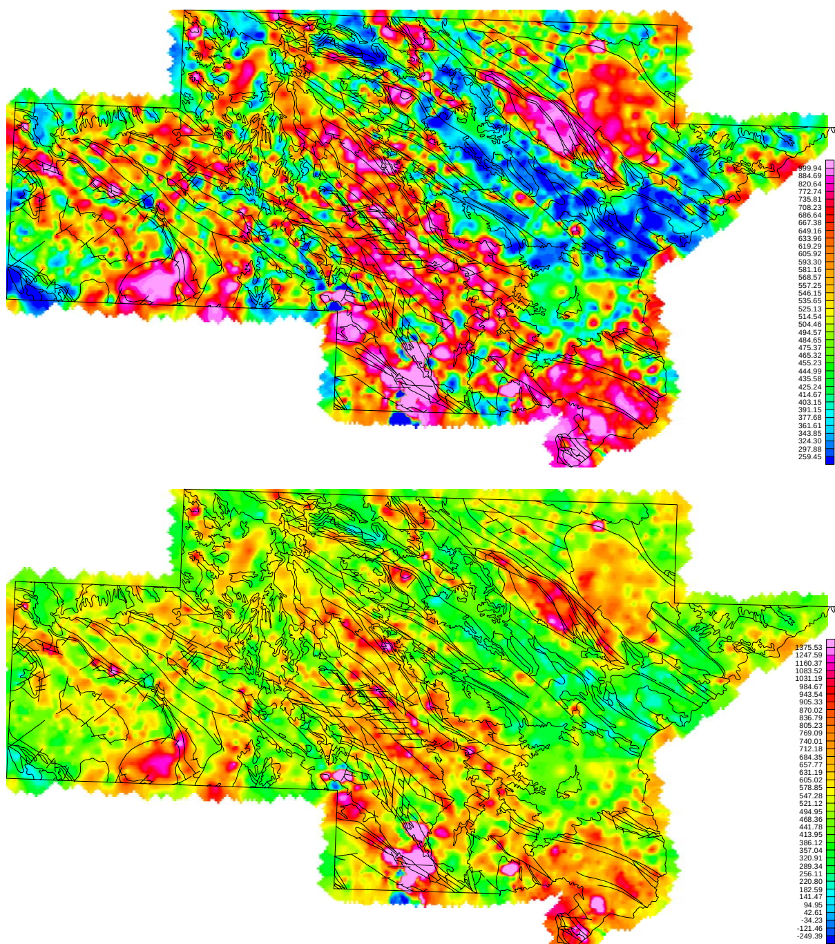
Figura 6-257. Mapas de distribución de Ba con escala ecualizada a partir del histograma y con escala de distribución normal (debajo)
