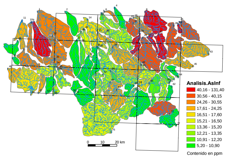
Figura 10-3. Mapas de distribución de contenidos de As en las muestras de techo y base de llanuras de inundación y del sedimento de corriente en el punto de desmuestre.
