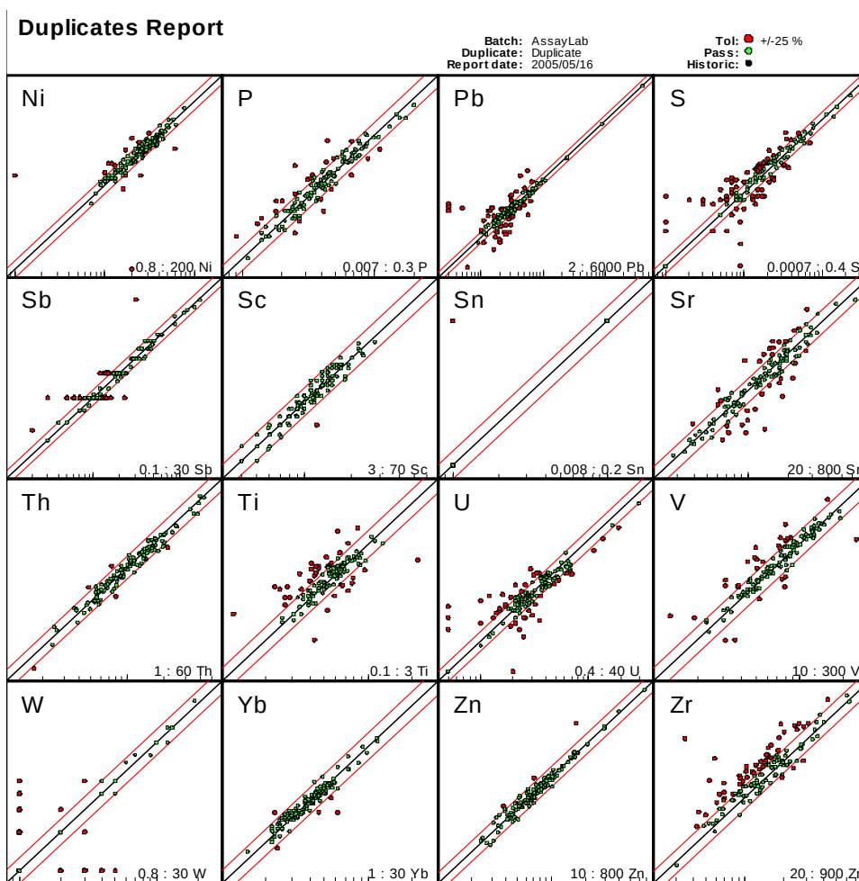
Figuras 6-6 a y b. Correlaciones entre las determinaciones analíticas en muestras y duplicados
