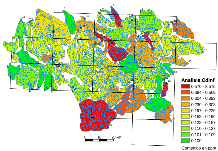
Figura 10-7. Mapas de distribución de contenidos de Cd en las muestras de techo y base de llanuras de inundación y del sedimento de corriente en el punto de desmuestre.
