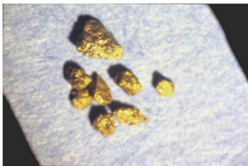
Foto 7-26. Granos de pirita sin oxidar. M-0761. 50 aumentos
