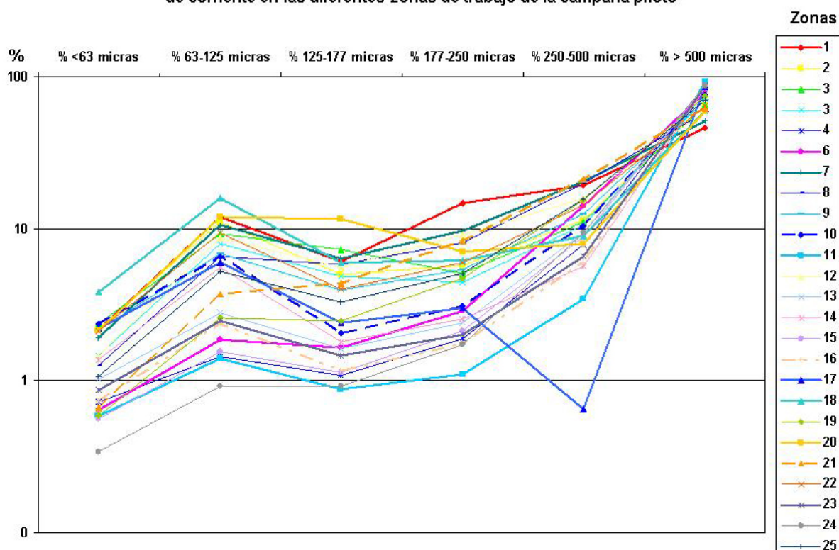
Figura 5-2 a. Variación porcentual del peso de las fracciones granulométricas de las muestras de sedimentos de corriente en las diferentes zonas de trabajo de la campaña piloto
