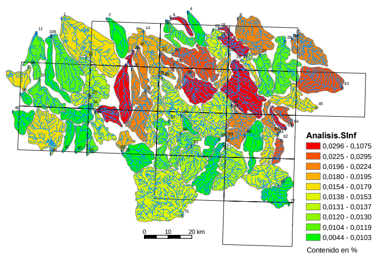
Figura 10-20. Mapas de distribución de contenidos de S en las muestras de techo y base de llanuras de inundación y del sedimento de corriente en el punto de desmuestre.
