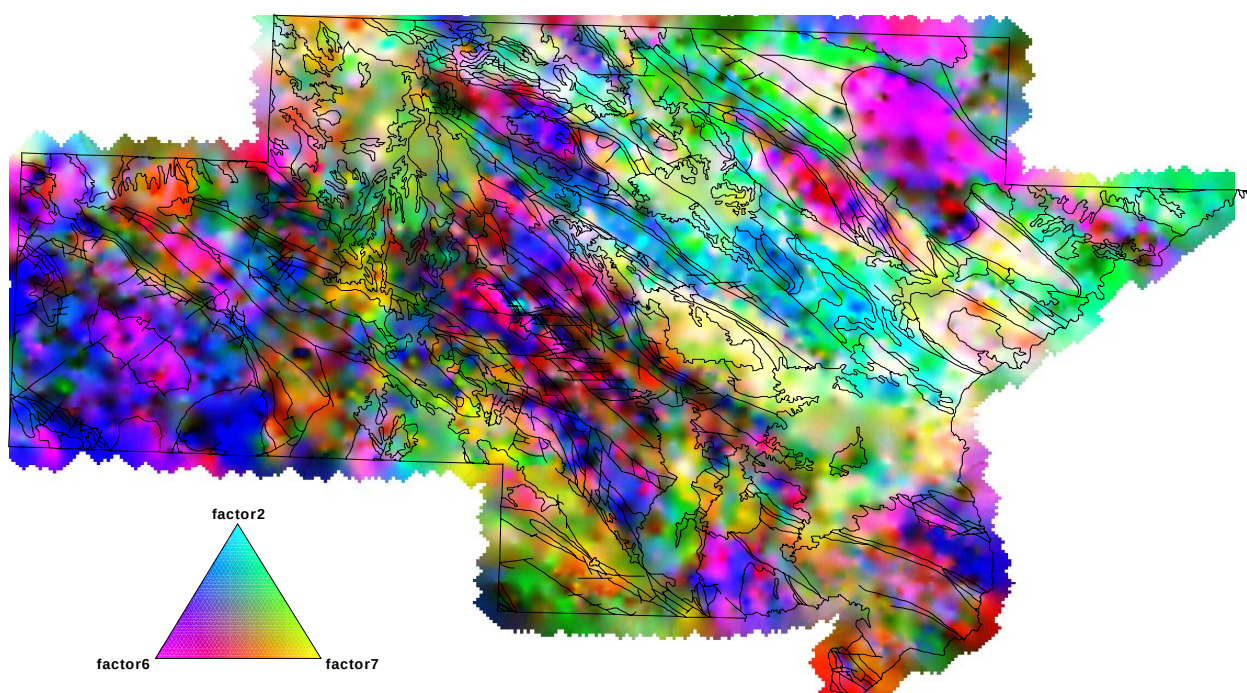
Figura 6-337. Mapa ternario CMY de F2-F6-F7
