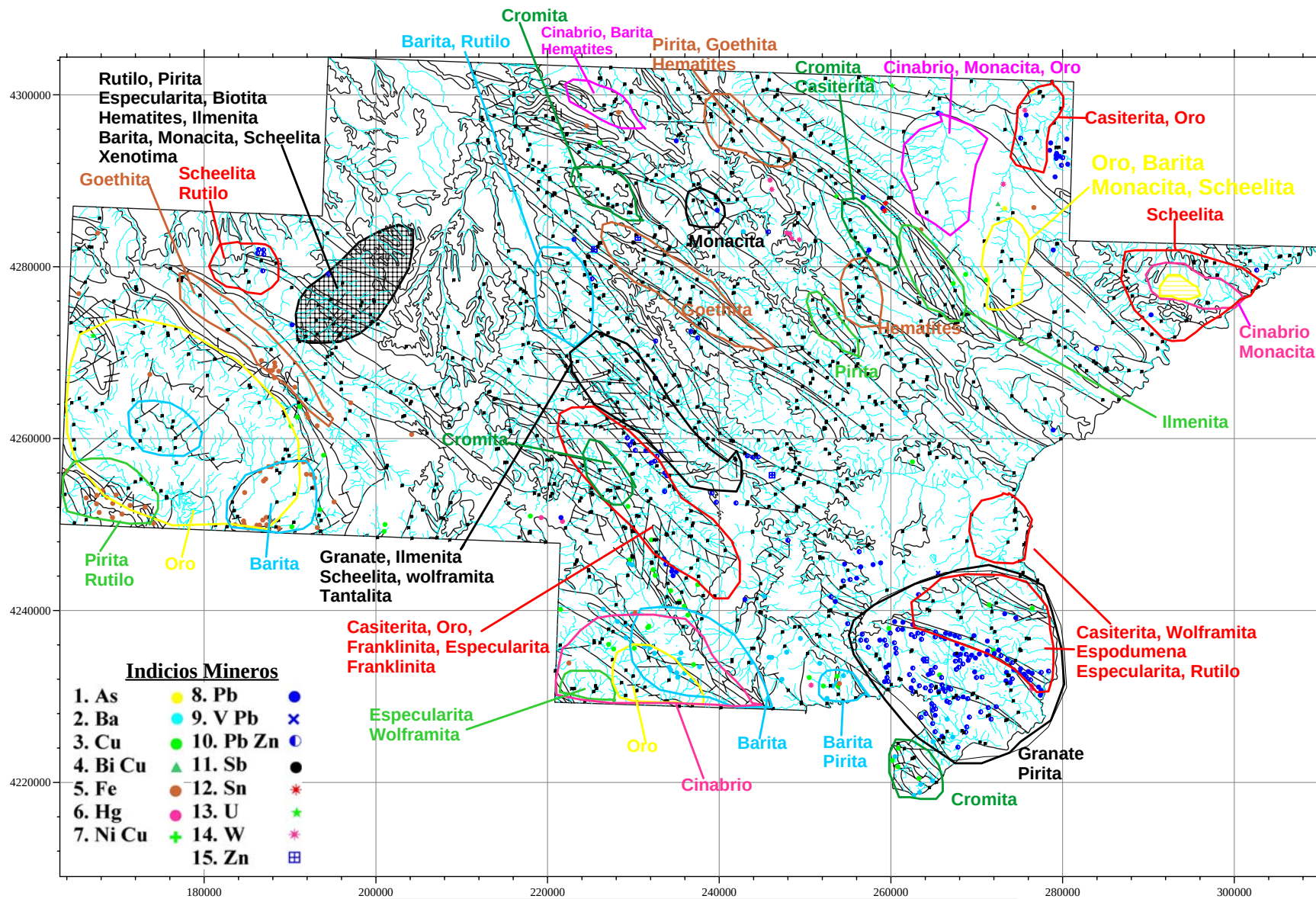
Figura 7-94. Esquema de síntesis de los rasgos de distribución de minerales pesados y de las principales anomalías minerlométricas.
