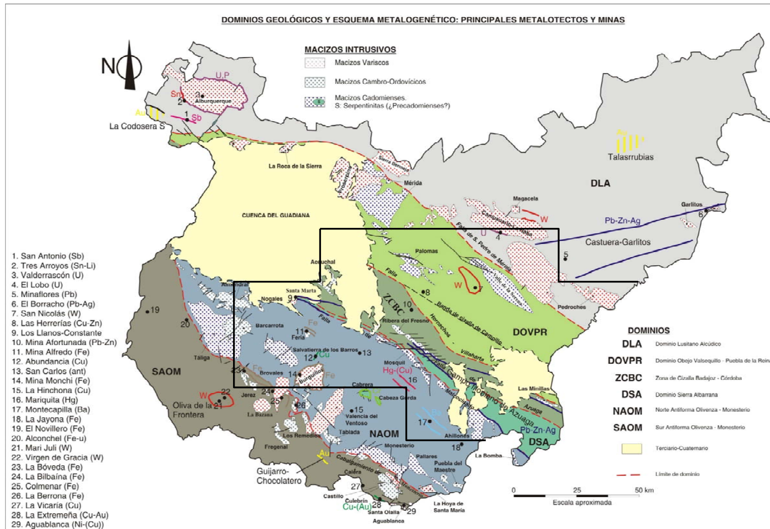
Figura 2-7. Esquema de dominios metálicos y principales metalotectos de la provincia de Badajoz. Fuente: Mapa Metalogenético a escala 1/200.000 de Badajoz (IGME-Junta Extremadura, 2 005)
