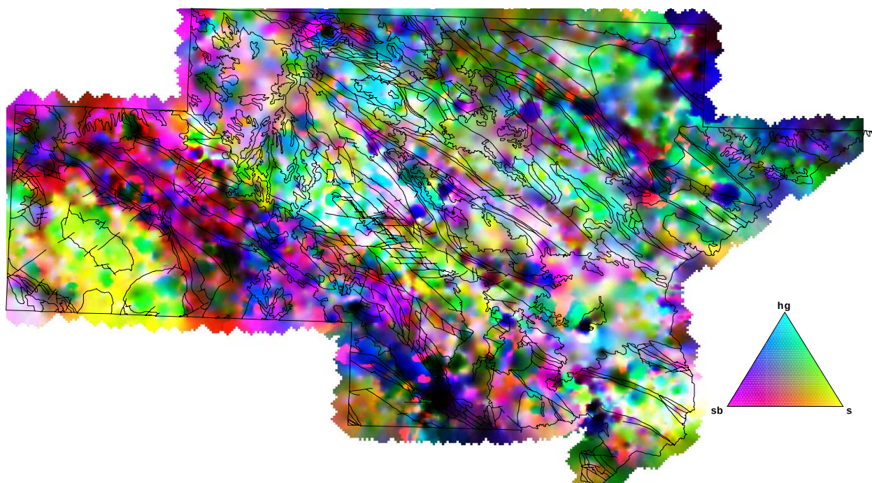
Figura 6-327. Mapa ternario CMY de Sb-Hg-S
