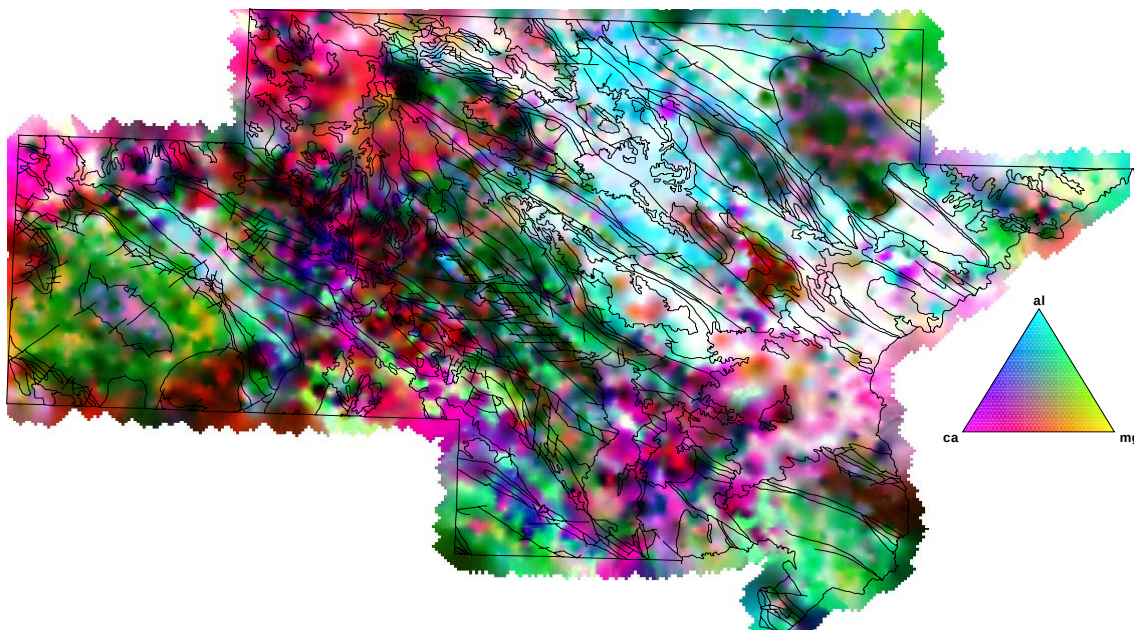
Figura 6-312. Mapa ternario CMY de Al-Ca-Mg
