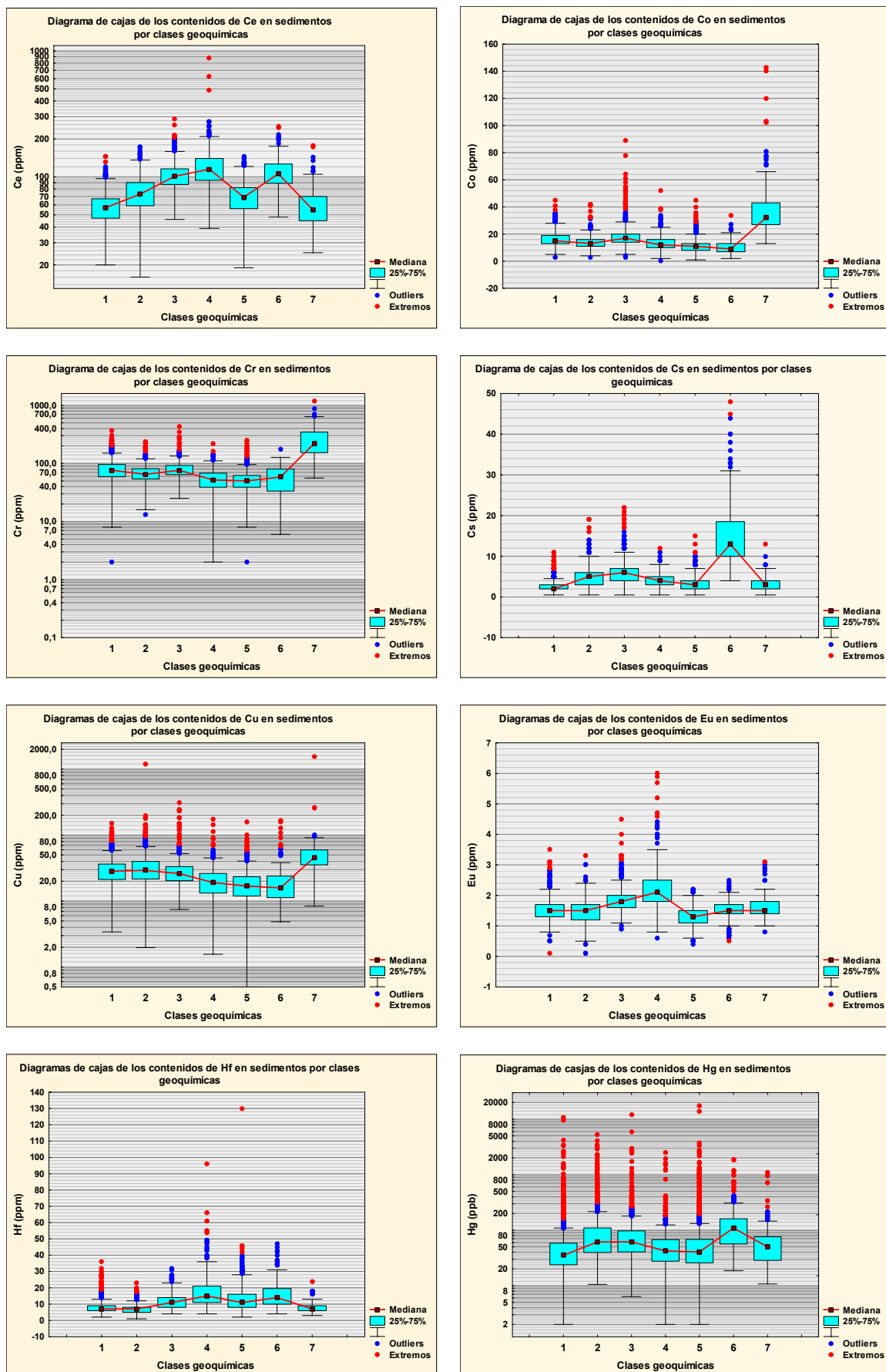
Figuras 6-362 a 6-369. Diagramas de cajas, por clases geoquímicas, de las concentraciones geoquímicas de elementos traza en sedimentos de corriente
