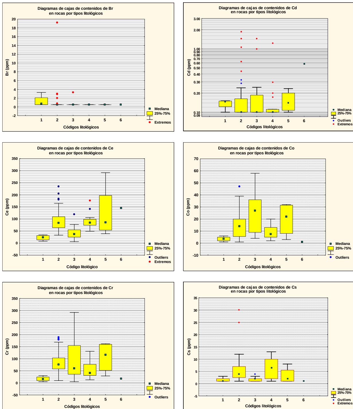
Figura 4-65 a 4-70. Diagramas de cajas de contenidos de elementos traza por tipos litológicos
