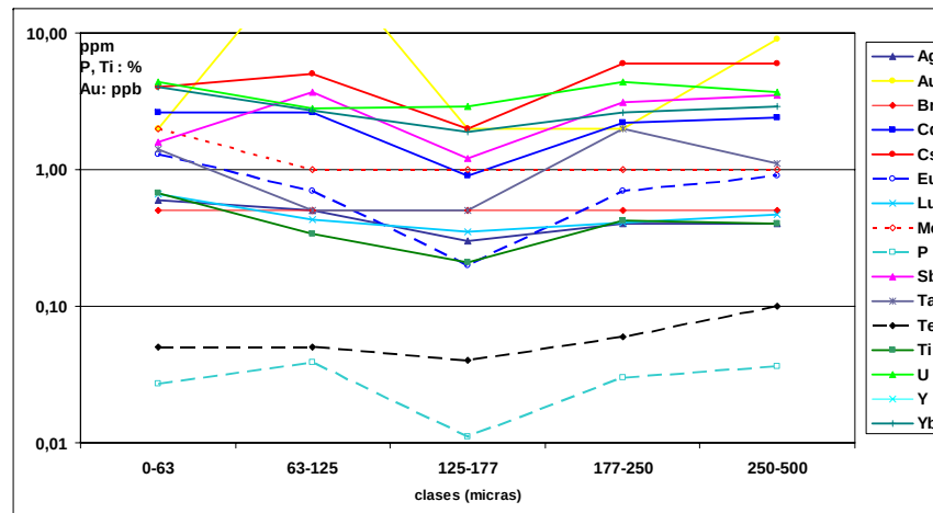
Figura 5-22 d. Zona 10 - Muestra 22 - Suelo. Variación de los contenidos de elementos en diferentes fracciones granulométricas.
