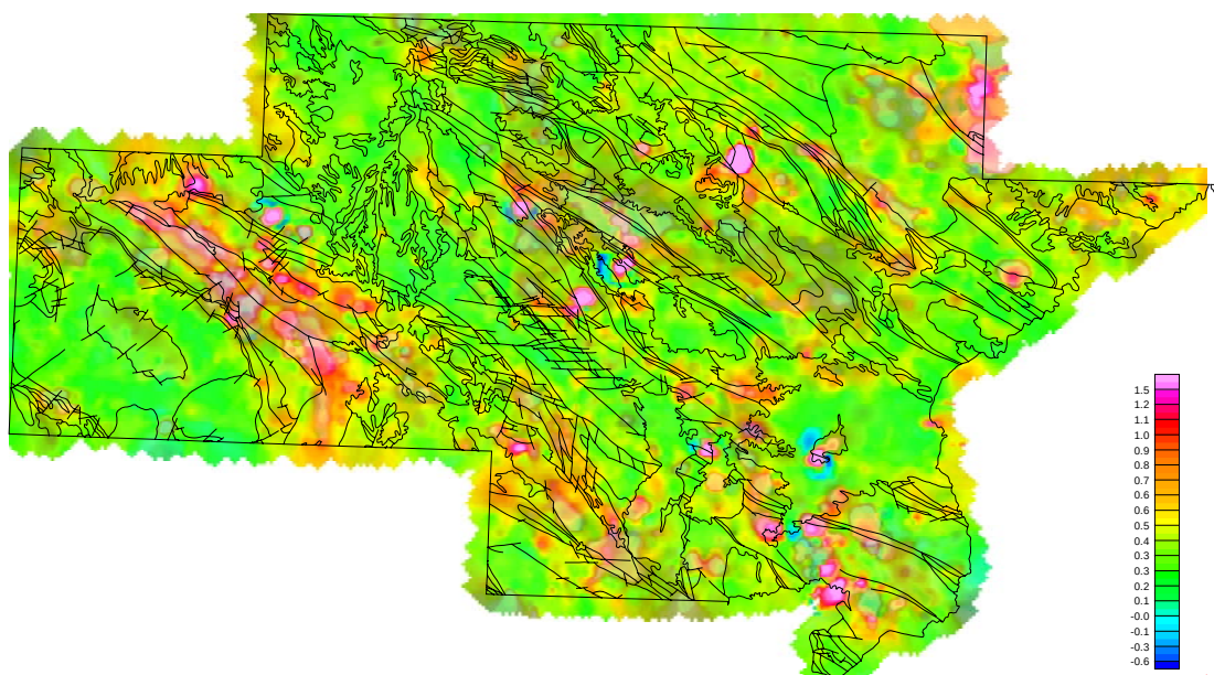
Figura 6-342. Mapa aditivo de Sb-Ag-Cd. Escala log-lineal
