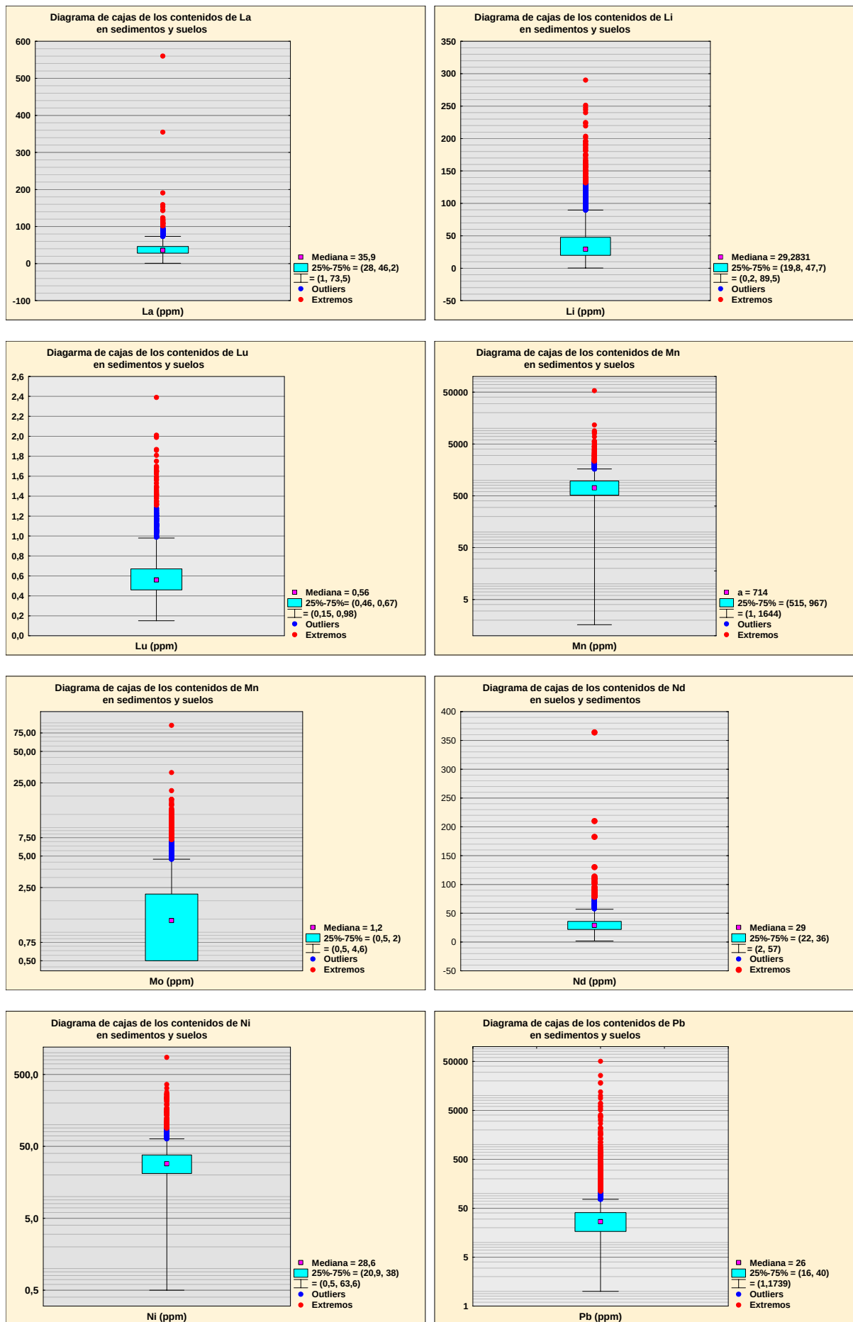
Figuras 6-81 a 6-88. Box Plots de concentraciones de elementos traza en la población muestral total
