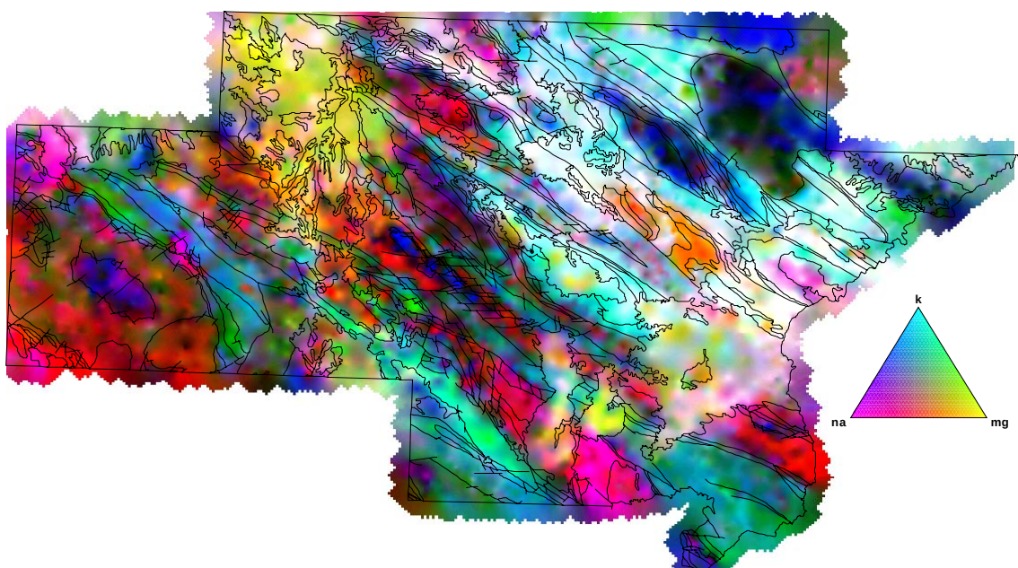
Figura 6-313. Mapa ternario CMY de Na-K-Mg
