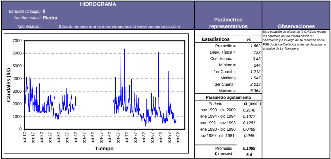
Figura 8. Análisis del hidrograma de la estación de aforo 8 (río Piedra)
