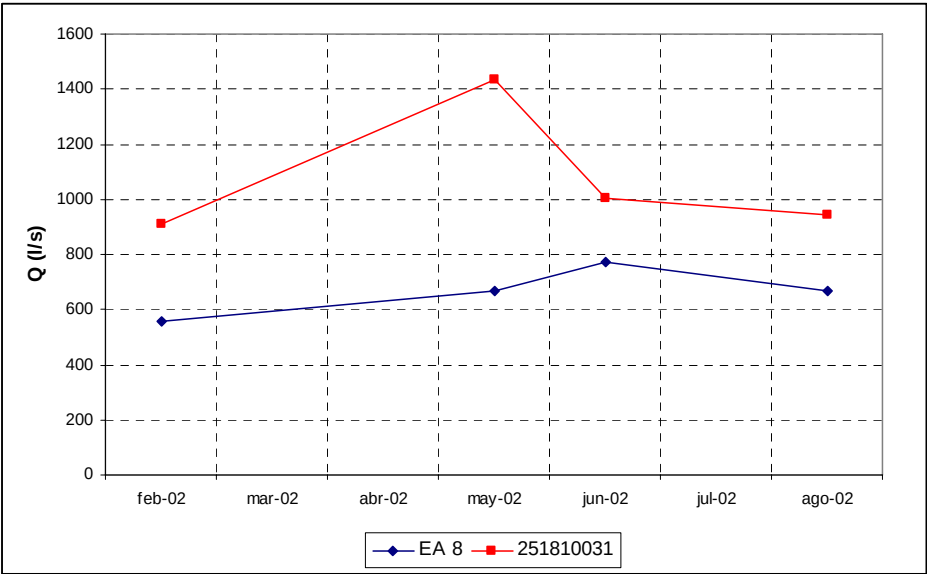
Figura 13. Aforo diferencial en el curso del río Piedra (año hidrológico 2001-2002)
