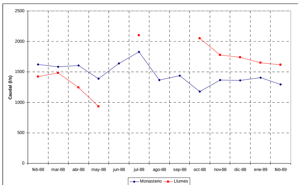
Figura 14. Aforo diferencial en el curso del río Piedra (año hidrológico 1988-1989)
