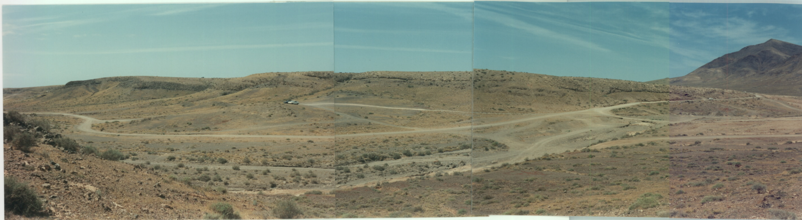
Fot. 9.- Panorámica del barranco que desciende a la Playa de las Mujeres. Alternancia de materiales piroclásticos alterados, coladas basálticas y coladas de traquitas máficas del tramo inferior del edificio Ajaches. Autor: J.A. Gómez
