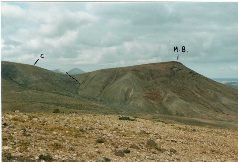
Fot. 27.- Panorámica de las laderas occidentales del edificio Montaña Bermeja (M.B.), discordante sobre las coladas basálticas miocenas (C).
