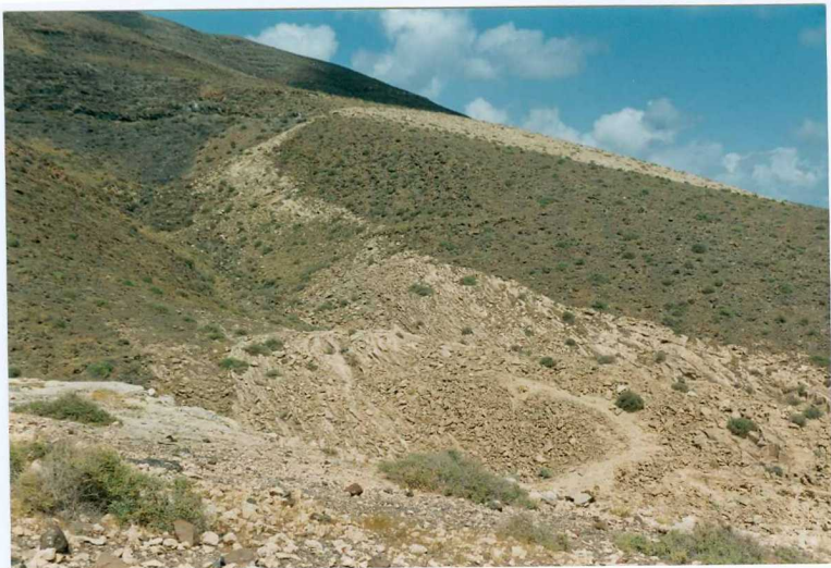
Fot. 21.- Arenas eólicas pliocenas adosadas a los relieves miocenos, al sur de los Morros de Hacha Chica.
