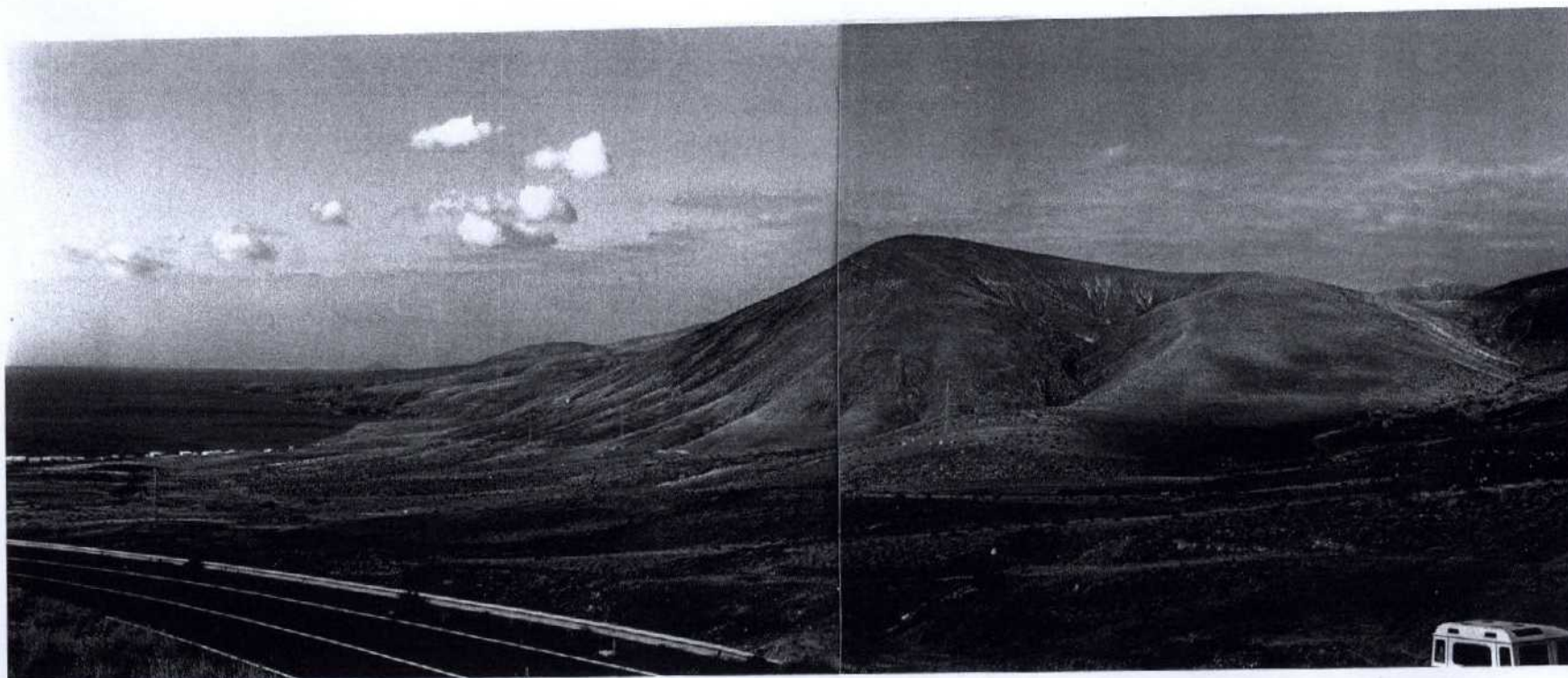
Fot. 26.- Panorámica del edificio Montaña Bermeja. A la izquierda se observa Playa Quemada y, al fondo, los relieves miocenos del Macizo de los Ajaches.
