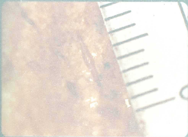
28-34 - FI-AN-3001.- Calcarenita con Lepidocyclinas (Oligoceno). (Sierra de la Horna).
