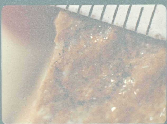
28-34-FI-AN-3005.- Calcarenita con Orbitolinas (Gil Martinez).
