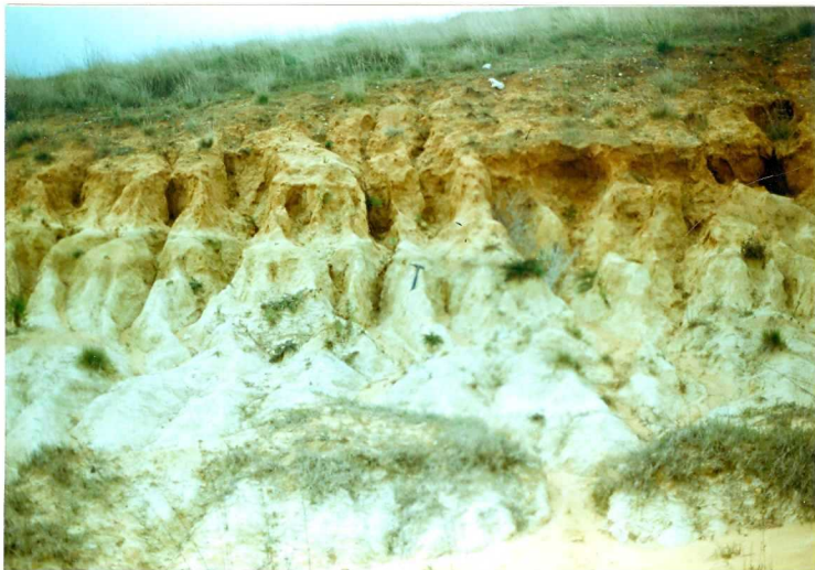
FOTO 25.- Niveles de arcillas y limos de la Facies Badajoz (Mioceno).
