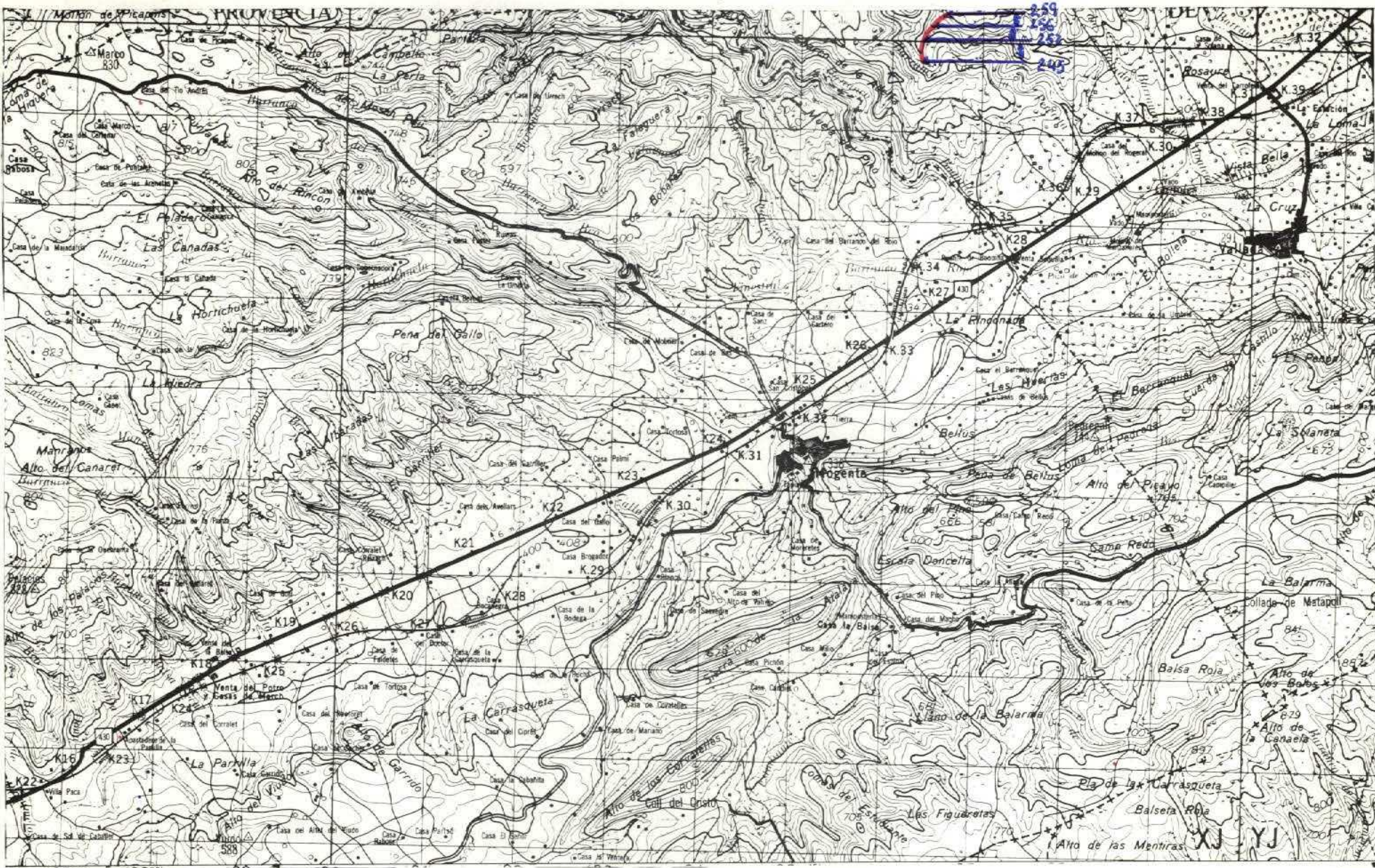
CORTA LA PERERETA (TRAMO I)
