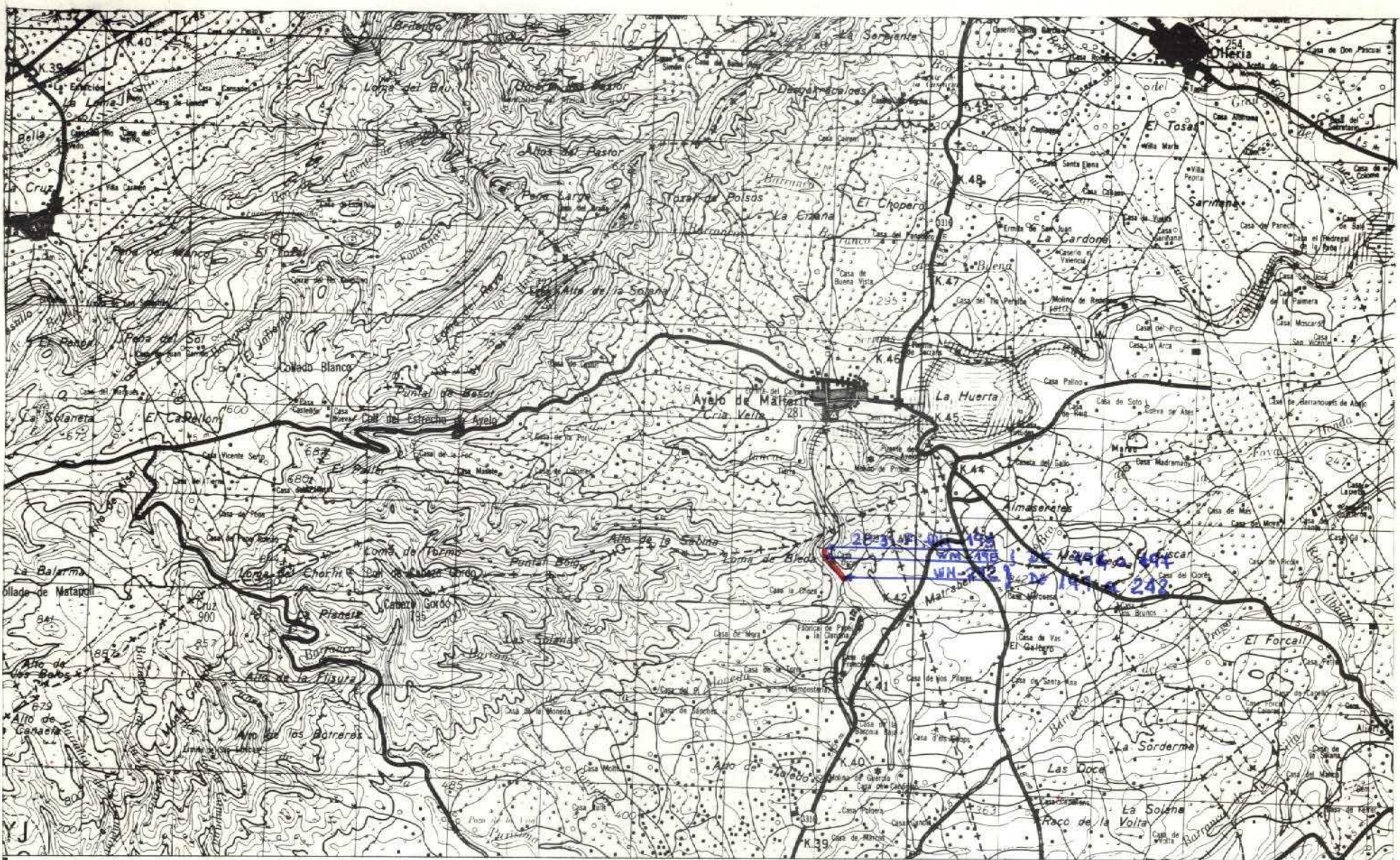
CORTE RIO CLARIANO
