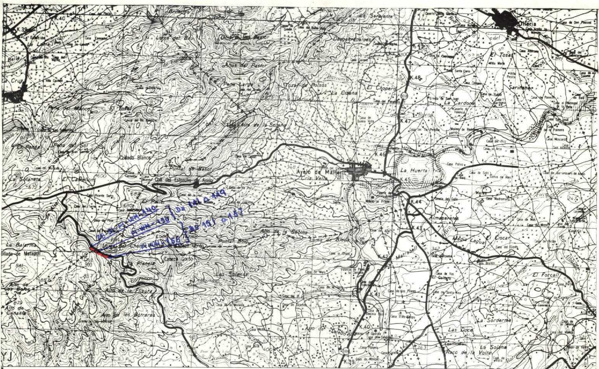
CORTE SIERRA GROSSA TRAMO A
