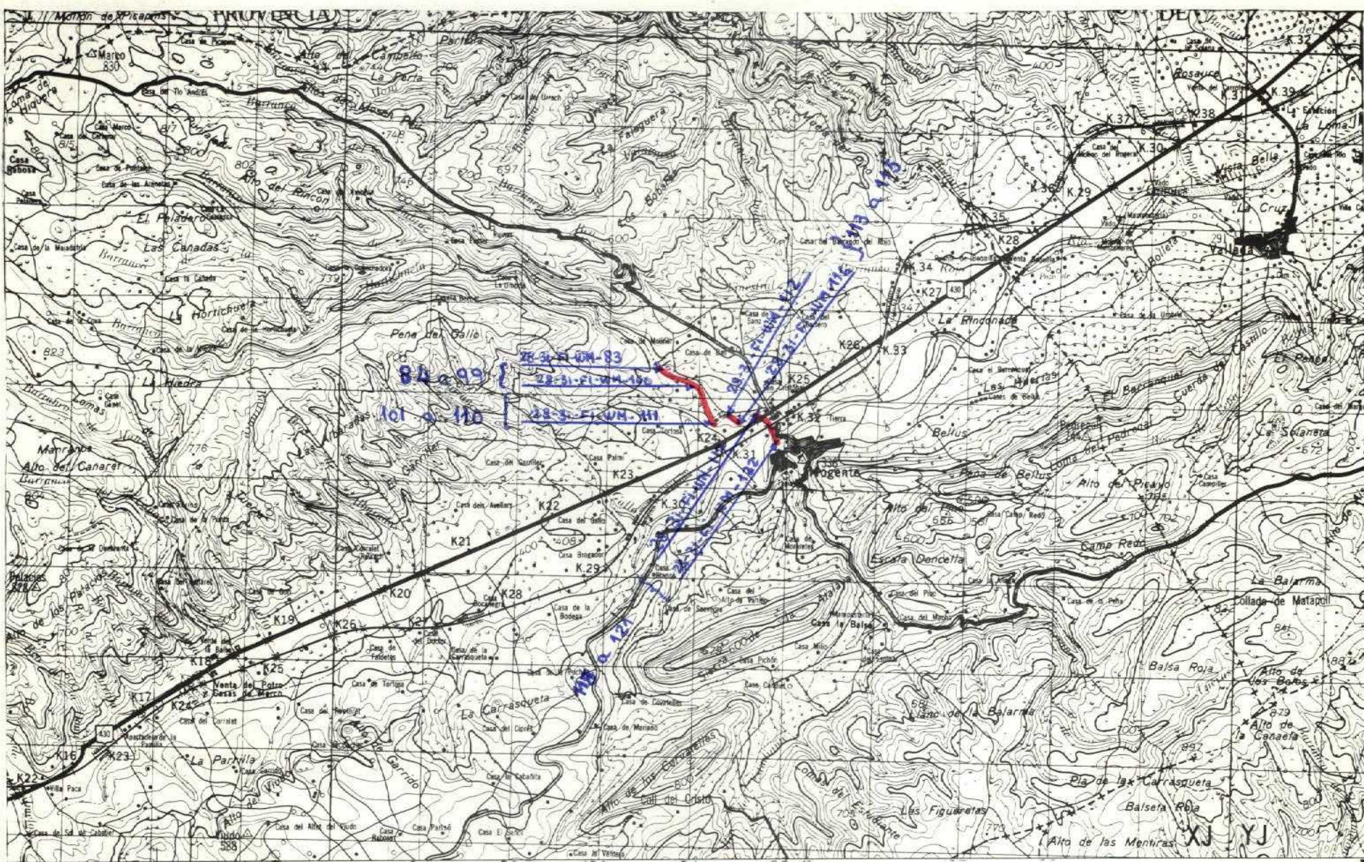
CORTE ESTRATIGRAFICO BARRANCO DE LA HOZ DE MOGENTE
