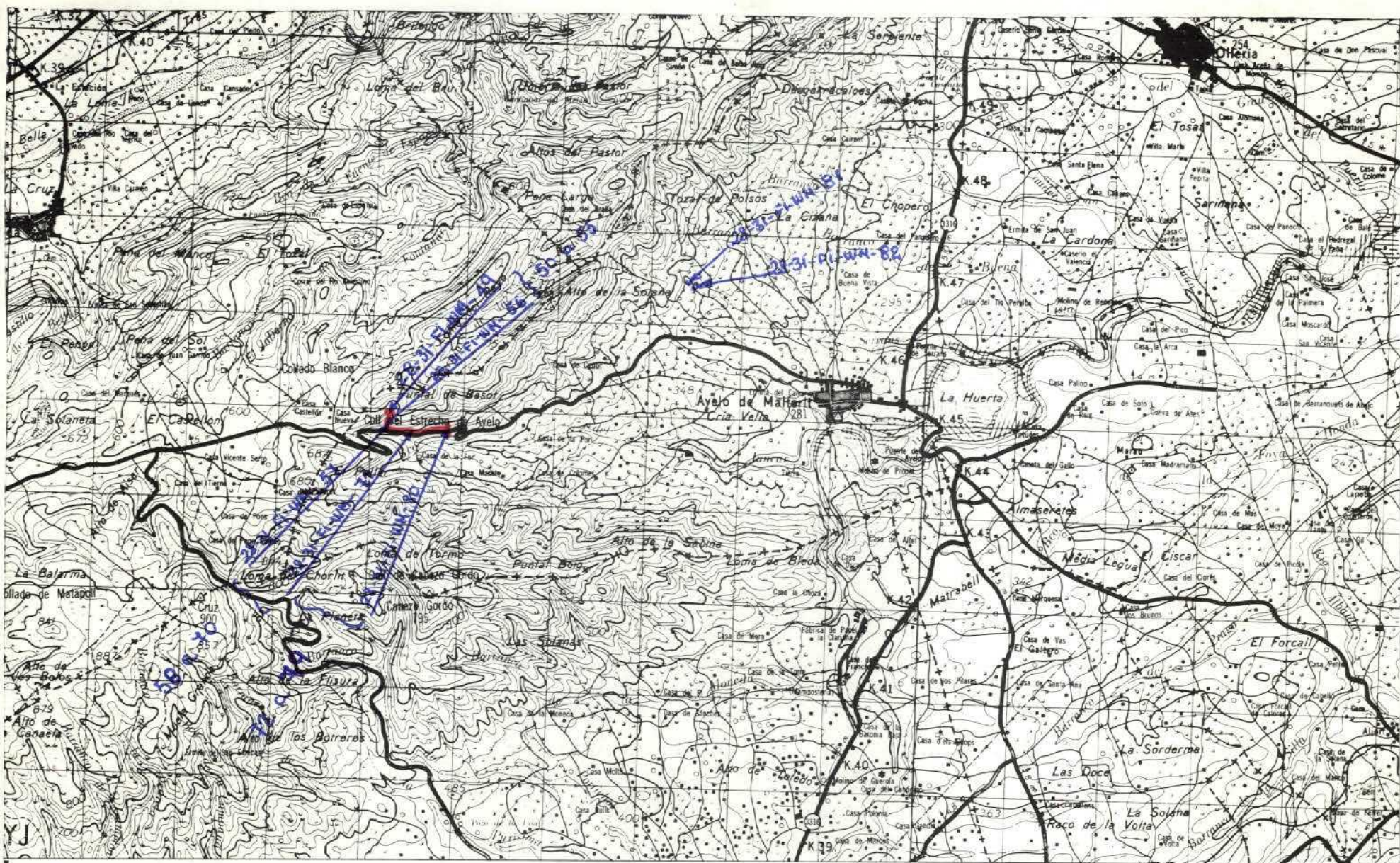
CORTE ESTRATIGRAFICO - COLL DEL ESTRECHO DE AYELO
