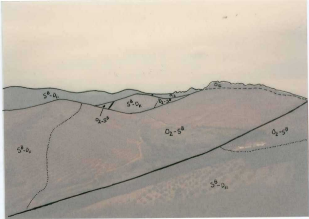
Foto nº 84.- Vista panorámica del Arenigiense ( O_{12} ), Ordovícico-Silúrico ( O_2-S^B ) y Silúrico-Devónico ( S^B-D_{11} ) en las proximidades del Portillo del Uniebro.
