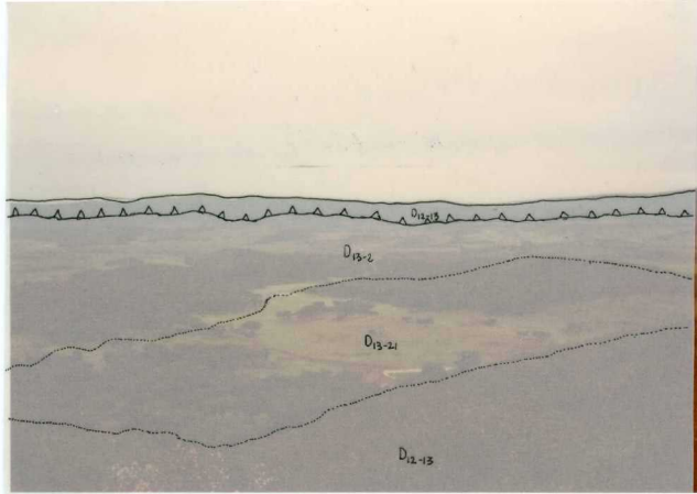
Foto nº 89.- Conjunto del Valle del Río Gévora. En primer término Siegeniense-Emsiense ( D_{12-13} ), cubierto por vegetación, luego calizas del Cobleciense superior - Eifeliense ( D_{13-21} ) y filitas del Gévora - ( D_{13-2} ); Al fondo cuarcitas del Siegeniense-Emsiense ( D_{12-13} ).
