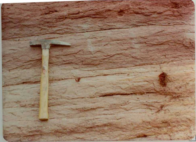
FM. 2137. Detalle del afloramiento representado en la fotografía anterior. (T G1-2 )
