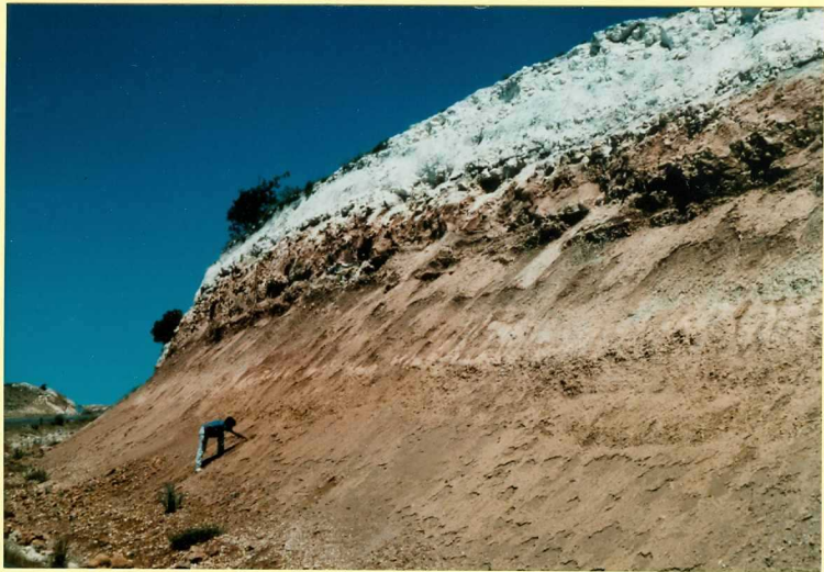
F-9108 Detalle del contacto entre las margocalizas somitales del Ciclo inferior del Páramo (unidad 8) y la Unidad detrítica basal del Ciclo superior del Páramo (9), al noroeste de Tórtoles de Esgueva Vallesense .
