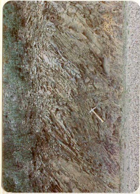
11-14-IB-VM-413.- Pliegue de arrastre (1ª Fase) en la secuencia turbidítica (W) en la carretera a las Torres de Aliste.
