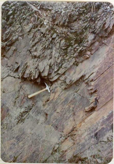
11-14/IB-VM-410.- Pliegue de 1 a Fase en el flanco norte de la secuencia turbidítica. (W).
