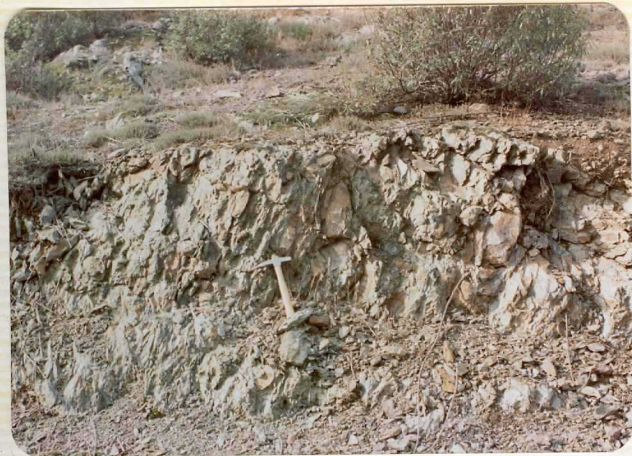
11-14/IB-VM-408.- Fanglomerado en las series Silúrico-Devónico, cerca de S. Blas (Carretera de Viñas a S. Blas).
