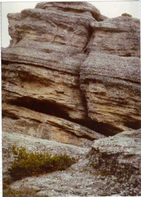
F-275. Conglomerado de la formación Urbión
