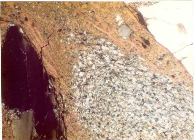
10-12-IB-JF 55 Crenulación en Ojo de Sapo cuarcítico LP, ob x 2, oc x 10
