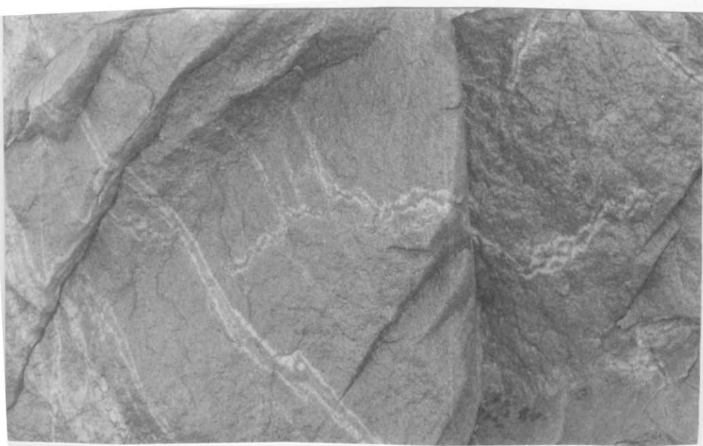
Estación 56. Hoja 03-12 (OYA) Microplegues de vanas de cuarzo en microgranitos biotíticos.
