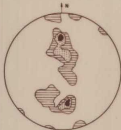
Diagrama de polos a planos S_1 (Estratificación) al N. de Viforcos: 26 polos. Curvas 3,5...9%
