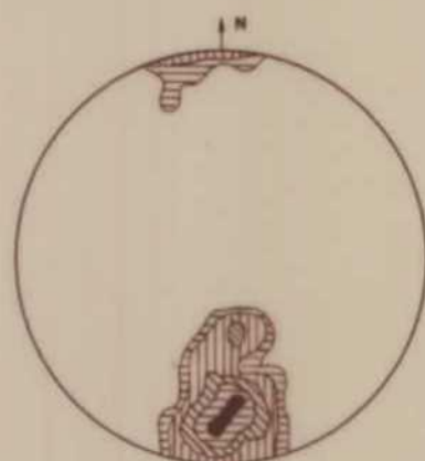
Diagramas de polos a planos S_2 (Esquistosidad) al N. de Brañuelas. 65 polos. Curvas 1, 3, 9, 15... 30%
