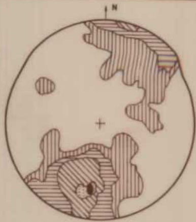
Diagrama de polos a S_1 (Estratificación) entre Malinaseca y Riego de Ambros 180 polos curvas 1,3... 15%
