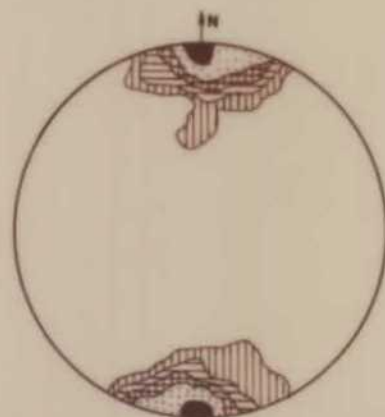
Diagrama de polos a planos S_2 (Esquistosidad) al O. de Viforcos. 72 polos Curvas 1, 3, 5, 11, 20 y 30%
