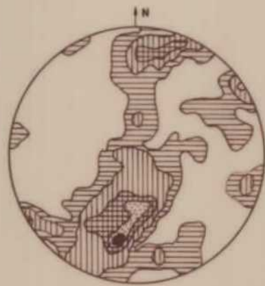
Diagrama de polos a planos S_1 (Estratificación) entre Santa Marina del Sil y Rodanillo: 73 polos Curvas 1, 3, 5... 10%
