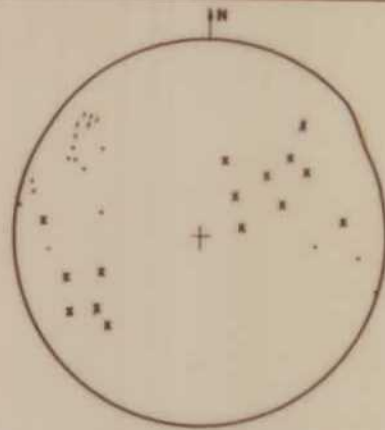
Ejes de la 1ª fase (-) y la 2ª fase (x) en el Cámbrico entre Malinaseca y Riego de Ambros
