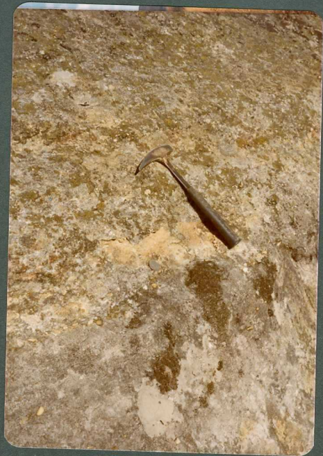
FOTO 5.- Areniscas conglomeráticas de la unidad C 1-1 15-21
