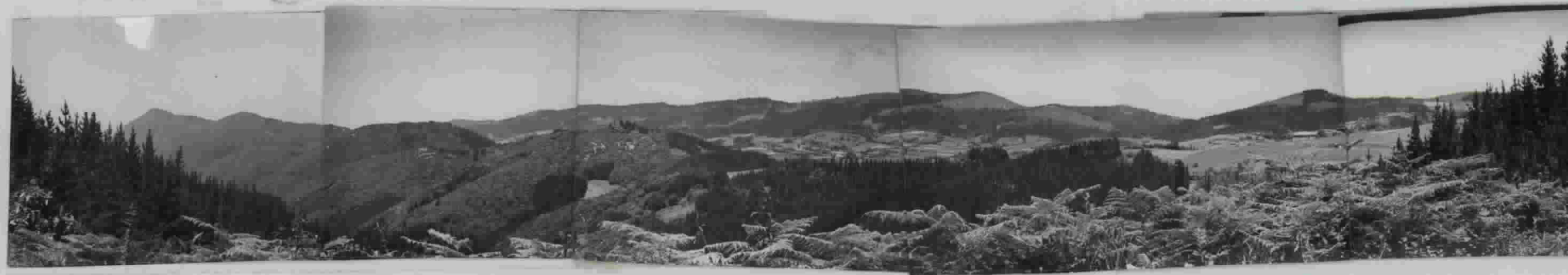
Fotos n os . 58 - 59 - 60 - 61 - 62.- Anticlinal de Navárniz (desde la entrada a Navárniz).
