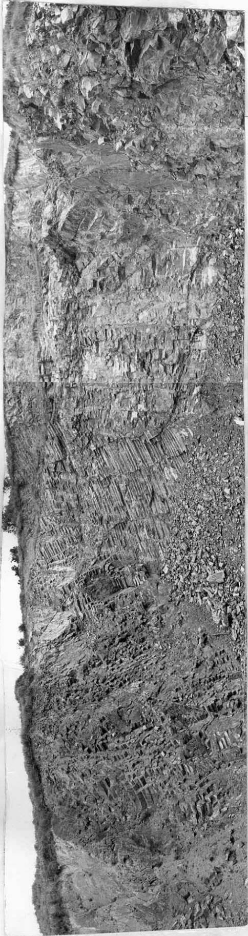
Fotos n os . 34 - 35 - 36. - Basalto (carretera de Frúniz a Gamiz Km 21-22)°.
