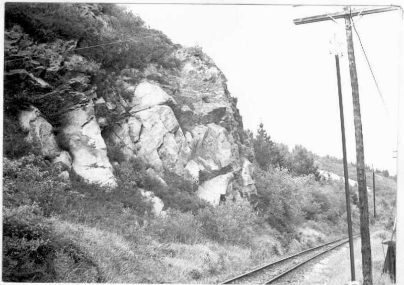
Foto nº 33. - Detalle de los crestones micro conglomeráticos de la base del flysch Danés-Ypresiense (carre tera Amorebieta - Guernica Km. 26).
