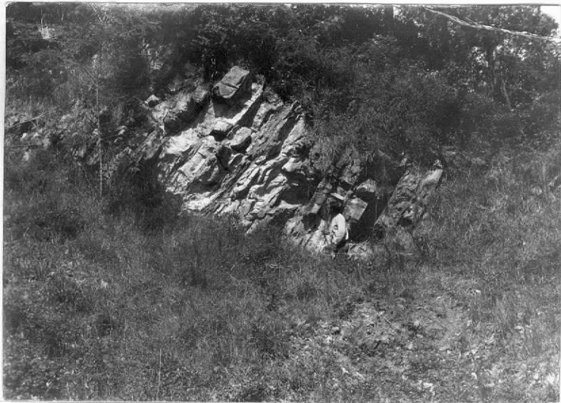
Foto nº 40 .- Aspecto de las calizas rojas del flysch Santoniense inferior Maas trichtiense (carretera de Marquina a Durango 43).
