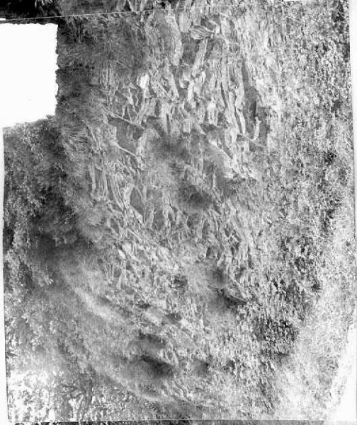
Fotos nºs 27 - 28 - 29.- Aspecto del flysch Danés-Ypresiense (carretera Amorebieta - Guernica Km 24).
