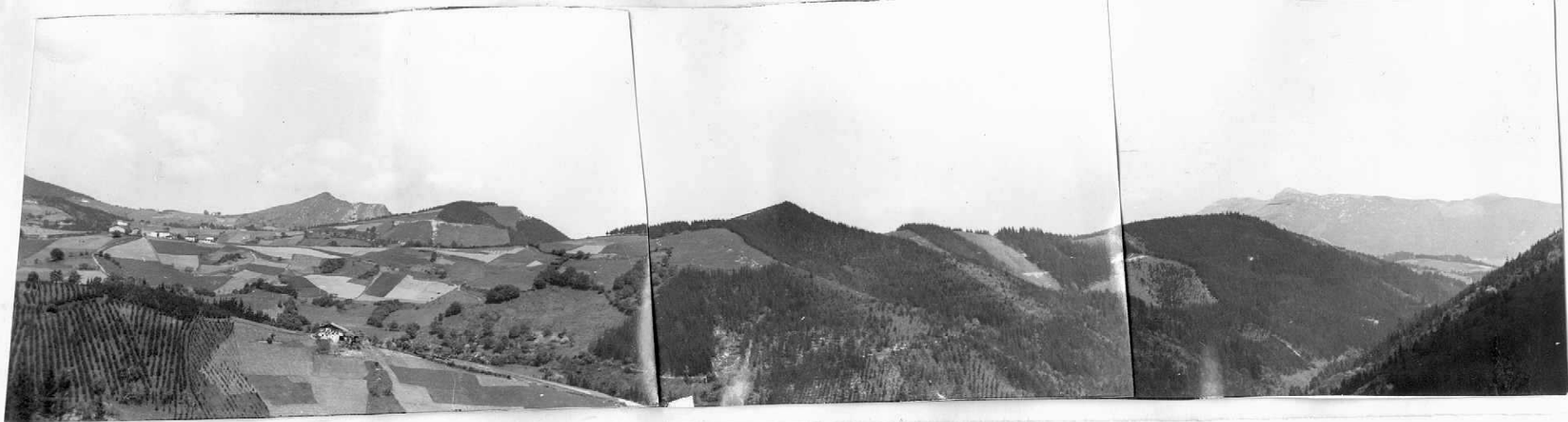
Fotos n os . 45 - 46 - 47 - 48. - En primer término el flysch Albiense - Santoniense inferior, al fondo las calizas del Aptiense - Albiense inferior (carretera Marquina a Du rango, en el cruce del desvío a Ermua).
