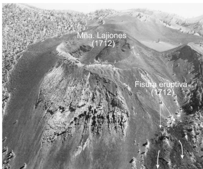
Fig. 2.18. Cono principal (Mña. Lajiones) y bocas efusivas más elevadas de la erupción de 1712. (Foto J.C. Carracedo).
