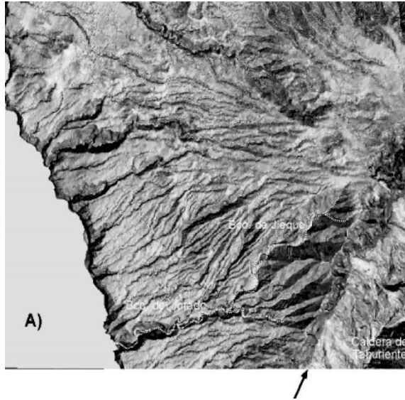
Fig. 2.19. Afloramiento del Edificio Garafia (flechas) en el fondo del Barranco de Jieque. Esta formación no aflora en la pared de La Caldera, a pesar de su proximidad, por hallarse entre este barranco y la pared el borde de colapso del Edificio Garafia.
