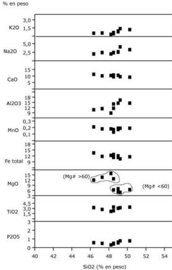
Fig. 5.17. Diagrama de variación de elementos mayores en lavas del edificio volcánico Garafia.
