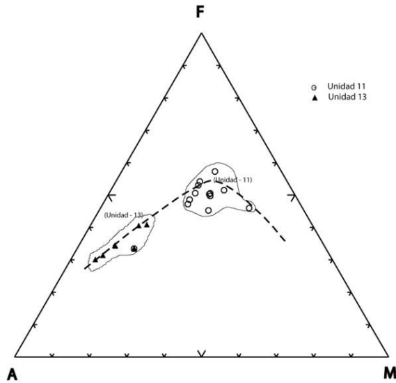
Fig. 5.28. Diagrama AFM del Edificio volcánico Taburiente superior.
