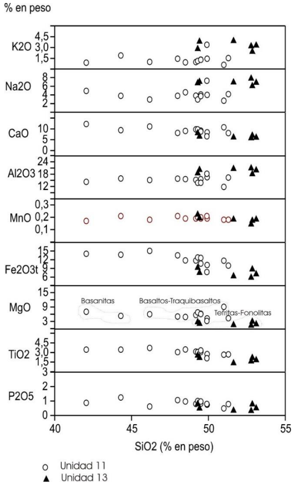
Fig. 5.29. Diagrama de variación de elementos mayores del Edif. Taburiente sup.
