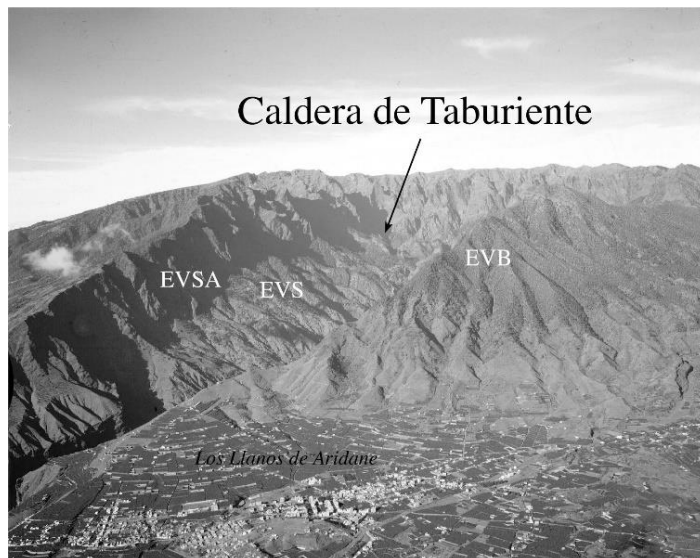
Fig. 2.9. Vista aérea oblicua de la Caldera de Taburiente. El cambio en la pendiente en las paredes de la caldera indica el tránsito del edificio submarino (EVS) a los edificios subaéreos (EVSA). La pared de la izquierda (en sombra) está formada por materiales del edificio volcánico Taburiente, mientras que la de la derecha es el edificio Bejenado (EVB), más joven. El Barranco de Las Angustias que las separa es el ensanchamiento erosivo de una falla asociada al deslizamiento gravitatorio de una de las dorsales del Taburiente (Dorsal o "rift" de Cumbre Nueva). Sobre la cuenca de este deslizamiento se formó, en discordancia, el Bejenado (Foto J. C. Carracedo).
