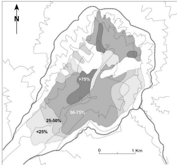
Fig. 2.15. Densidad de diques (en %) intruyendo en el fondo de la Caldera de Taburiente.
