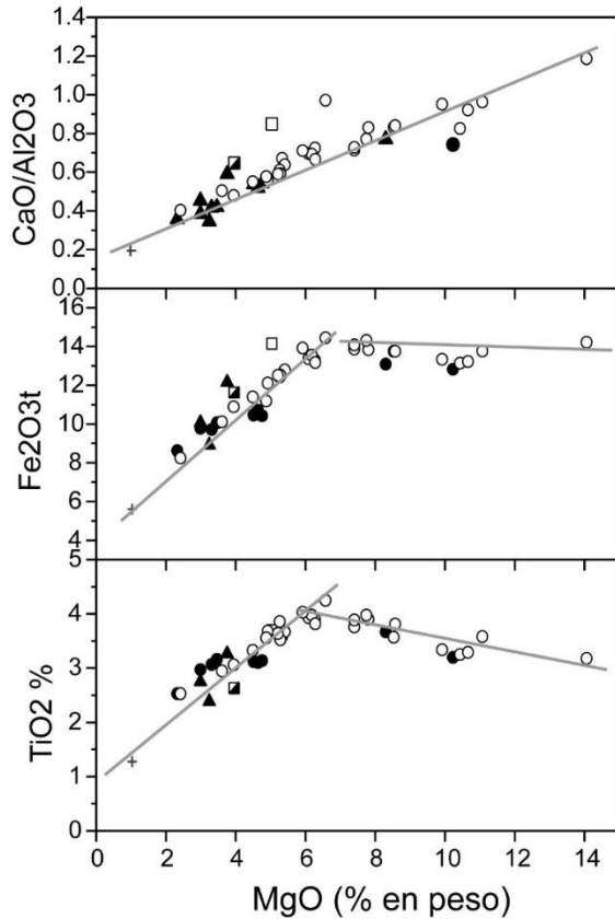
Fig. 5.36. Diagrama de variación de CaO/Al 2 O 3 y de elementos ferromagnesianos frente a los contenidos en MgO del edificio volcánico Bejenado. Símbolos como en la Fig. 5.33.
