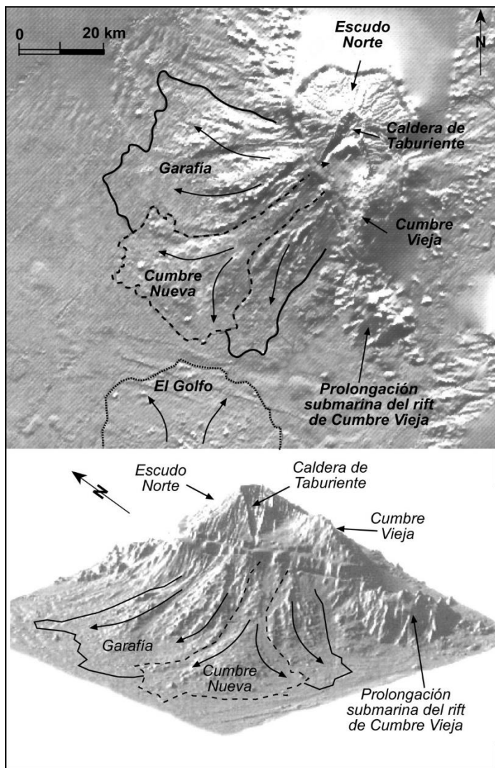
Fig. 3.2. Imágenes en relieve sombreado mostrando la extensión de los deslizamientos de Garafía y Cumbre Nueva. La dorsal ("rift") de Cumbre Vieja, la Caldera de Taburiente y el "rift" submarino continuación del de Cumbre Vieja se ponen como referencia. Se aprecia claramente cómo los materiales deslizados de Cumbre Nueva se asocian con el Barranco de Las Angustias y el arco de Cumbre Nueva, que son los límites del bloque desgajado (Imágenes de Urgelés, 1999).
