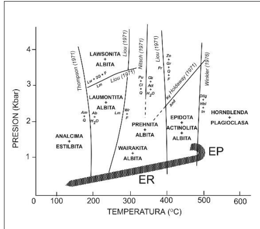
Fig. 2.13. Paragénesis minerales originadas en procesos de metamorfismo hidrotermal en la formación submarina del fondo de la Caldera de Taburiente.
