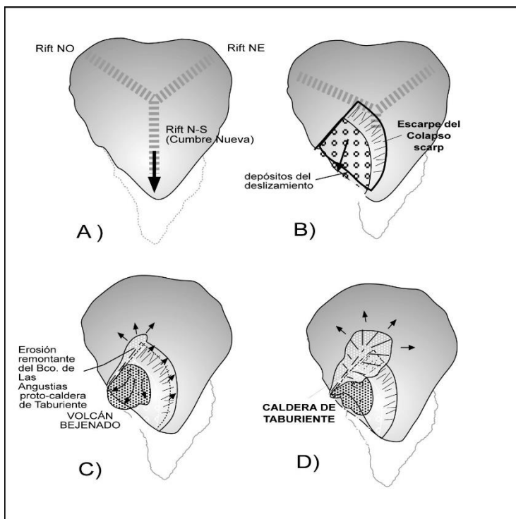
Fig. 3.4. Relación entre el deslizamiento de Cumbre Nueva y la formación de la Caldera de Taburiente (explicación en el texto).
