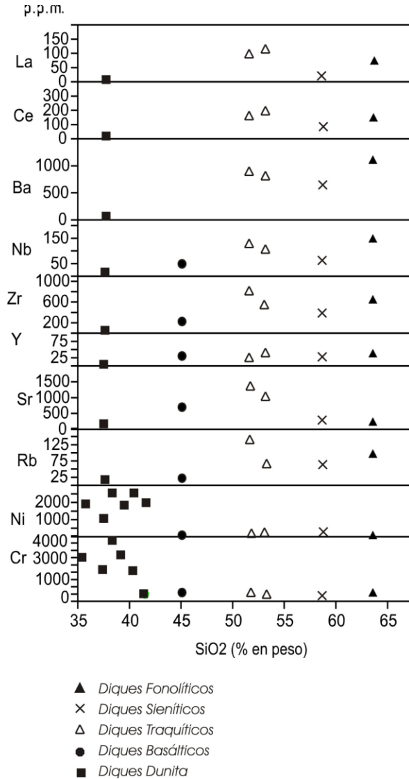
Fig. 5.13. Diagrama de variación de elementos menores de las intrusiones filonianas del Edificio Volcánico Submarino.
