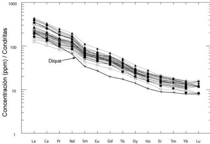
Fig. 5.38. Concentraciones de REE normalizadas-condritas de los materiales lávicos del edificio volcánico principal del Bejenado. Símbolos como en la Fig. 5.33.
