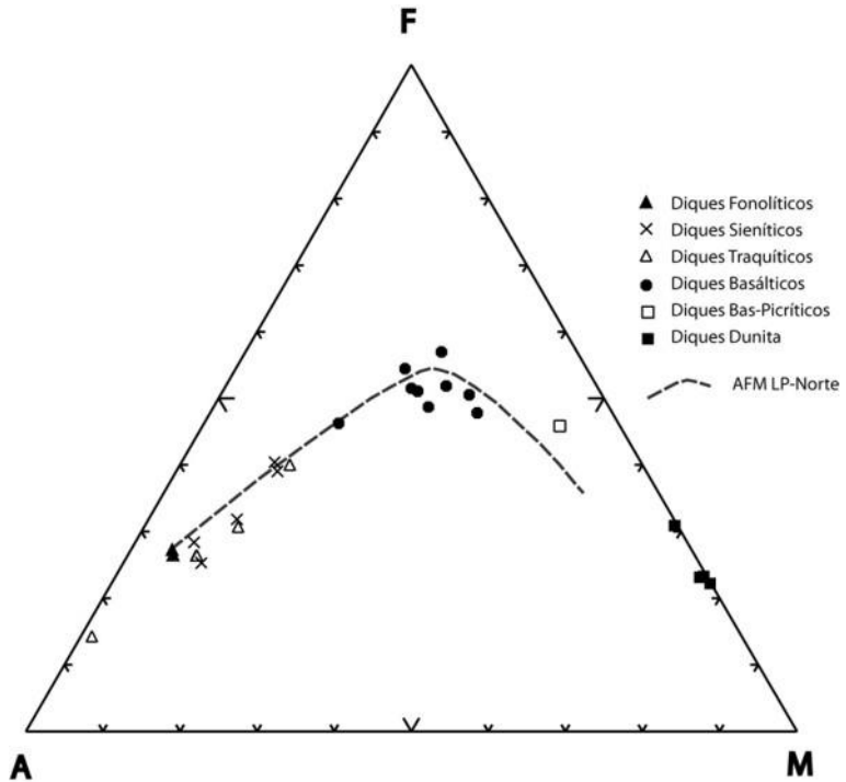
Fig. 5.11. Diagrama AFM de las Intrusiones filonianas del Edificio Volcánico Submarino.
