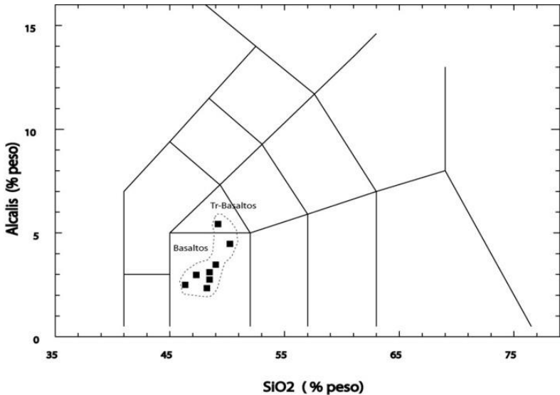
Fig. 5.15. Diagrama T.A.S. del edificio volcánico Garafia.
