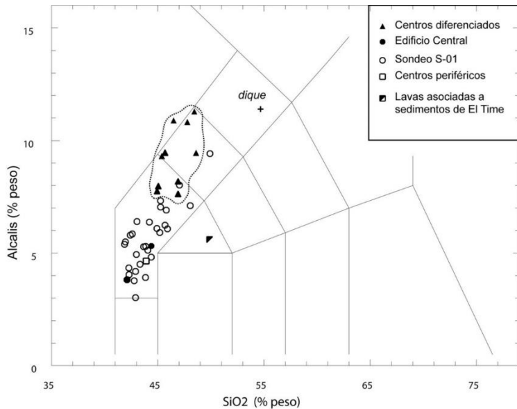
Fig. 5.33. Diagrama TAS del Edificio volcánico Bejenado
