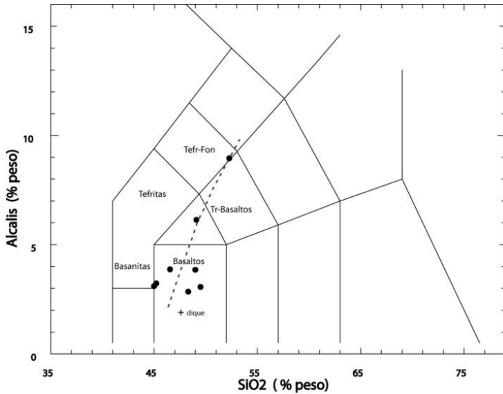
Fig. 5.21. Diagrama T.A.S. del edificio volcánico Taburiente Inferior.
