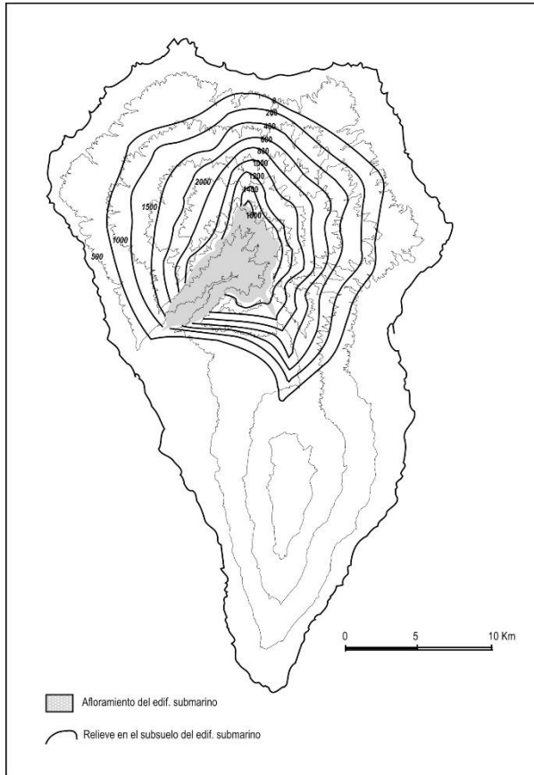
Fig. 2.8. Mapa esquemático indicando el afloramiento del edificio submarino en el interior de la Caldera de Taburiente y la extensión aproximada de esta formación submarina en el subsuelo de la isla (Coello, 1987).
