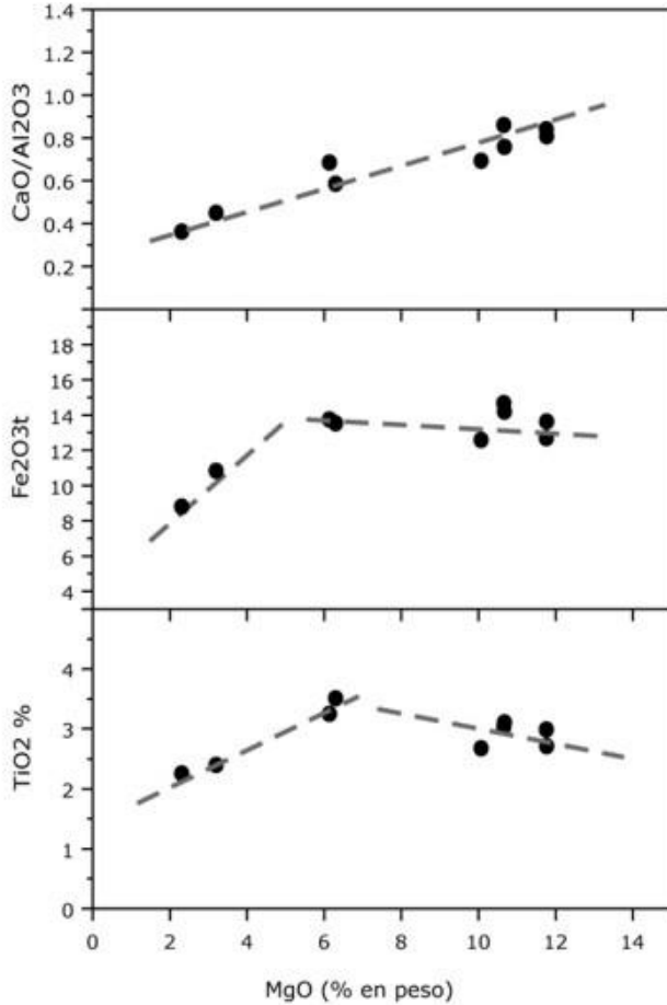
Fig. 5.24. Diagrama de variación de las relaciones \text{CaO}/\text{Al}_2\text{O}_3 , y de elementos ferromagnesianos frente al contenido en MgO del Edificio volcánico Taburiente inferior
