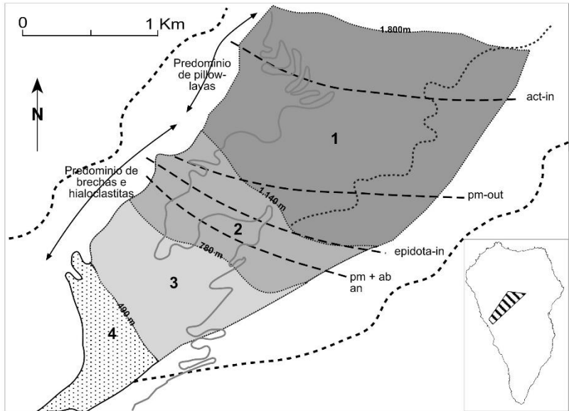
Fig. 2.11. Separación en cuatro secciones de la secuencia extrusiva submarina del fondo de la Caldera de Taburiente realizada Staudigel y Schmincke (1984). 1) Facies efusiva profunda. 2) Facies efusiva intermedia, con depósitos de flanco del monte submarino. 3) Facies efusiva intermedia a somera. 4) Facies volcanoclástica muy somera.
