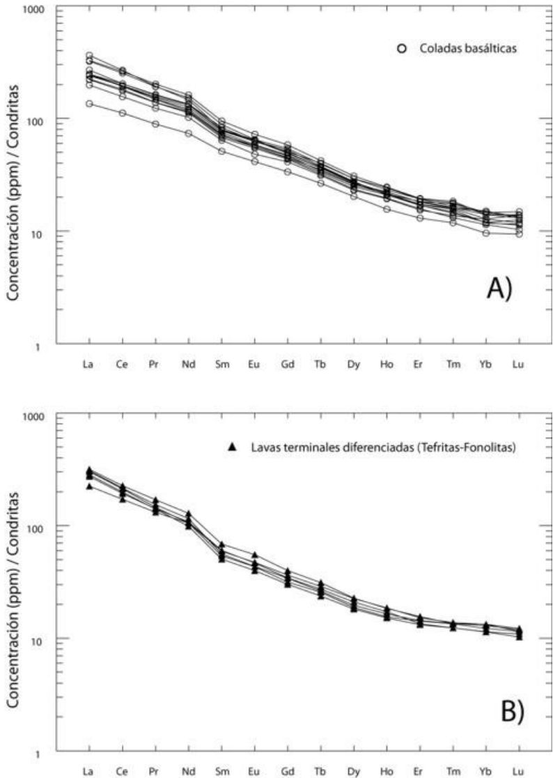
Fig. 5.32. Concentraciones de REE normalizadas-condritas del Edificio Volcánico Taburiente superior.
