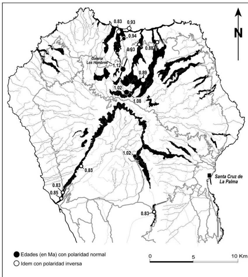
Fig. 2.21. Afloramientos del Edificio Taburiente Inferior. Los afloramientos de este edificio, al igual que el Edificio Garafia (infrayacente), se localizan en las cabeceras y cauces de los barrancos más profundos y en la base de la pared de la Caldera de Taburiente y el arco de Cumbre Nueva. En el primer caso son ventanas erosivas; en el segundo, estructuras tectónicas profundizadas por la erosión subsiguiente.
