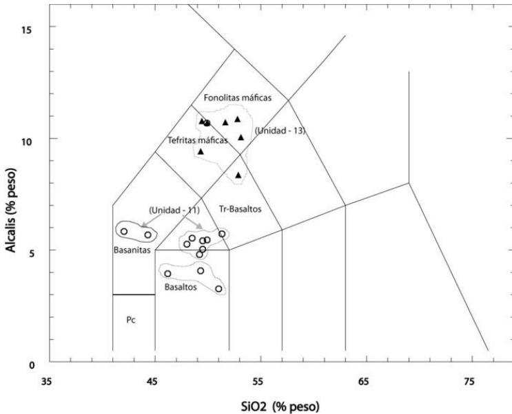
Fig. 5.27. Diagrama TAS del Edificio volcánico Taburiente superior
