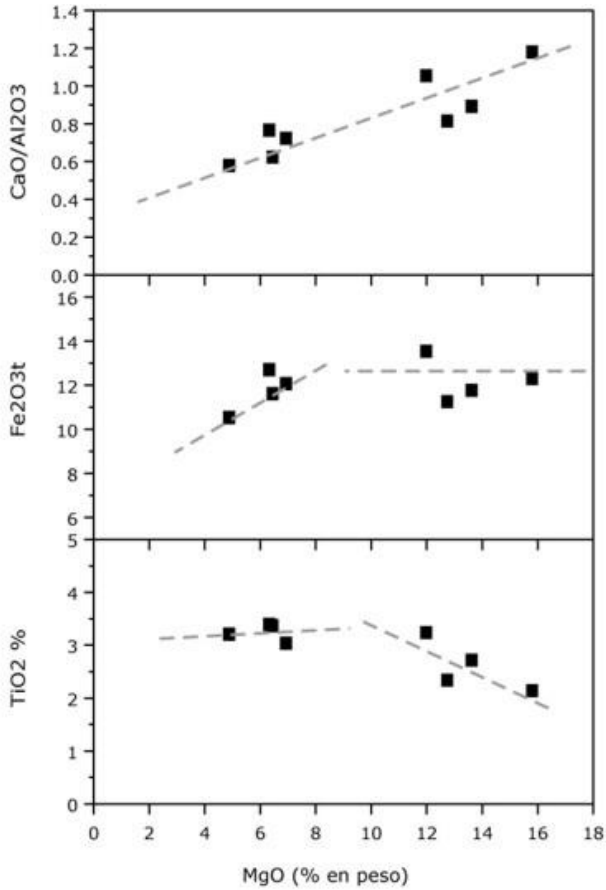
Fig. 5.18. Diagrama de variación de \text{CaO}/\text{Al}_2\text{O}_3 y de elementos ferromagnesianos frente a los contenidos en \text{MgO} del edificio volcánico Garafia.
