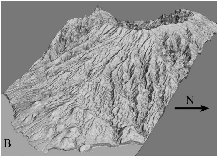
Fig. 2.25. B) El "rift" de Puntallana es un excelente ejemplo de la reorganización en "rifts" del Taburiente Superior. Imagen 3D a partir del mapa digital del IGN.
