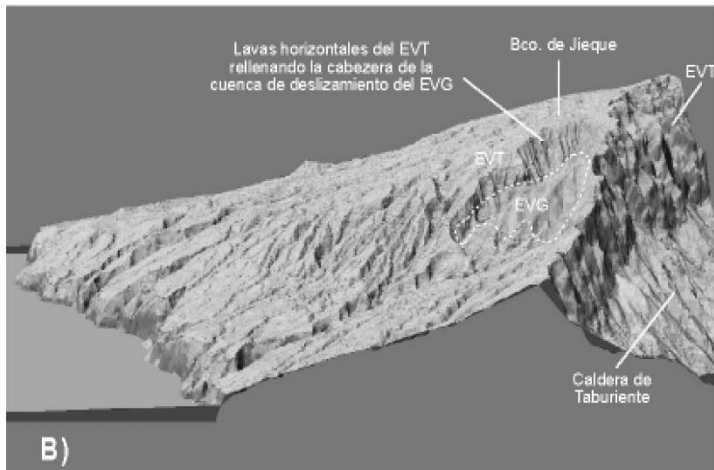
Fig. 2.20. Detalle de los afloramientos del Edificio Garafia en el fondo del Barranco de Jieque.
