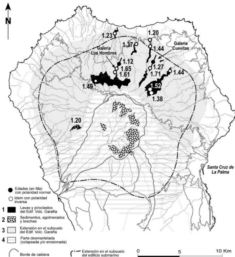
Fig. 2.16. Afloramientos del edificio volcánico Garafia (en negro). Se indica la extensión aproximada (deducida de observaciones en galerías) de este edificio volcánico en el subsuelo. Se aprecia claramente el flanco meridional desgajado (rayado) en el deslizamiento que afectó a este edificio hace 1.2 Ma. Se indica, como referencia, el contorno del edificio submarino. La formación sedimentaria que aflora en el interior de La Caldera (punteado) puede ser debida en gran parte al deslizamiento y erosión del Garafia.
