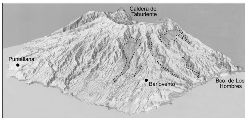
Fig. 2.17. Imagen del Norte de La Palma obtenida procesando las hojas digitales del IGN. Se ven los barrancos profundos donde aflora el edificio Garafia (en trama transparente).
