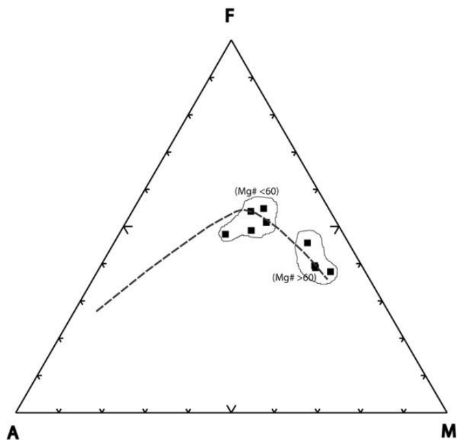
Fig. 5.16. Diagrama AFM del edificio Garafia.
