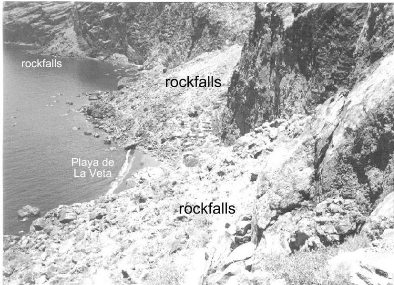
Fig. 2.28. Desplomes costeros ("rockfalls) de la Playa de La Veta (Foto J. C. Carracedo).
