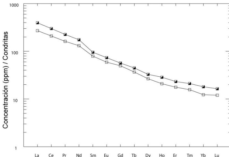
Fig. 5.39. Concentraciones de REE normalizadas-condritas de los materiales lávicos de los centros periféricos del edificio volcánico Bejenado. Símbolos como en la Fig. 5.33.
