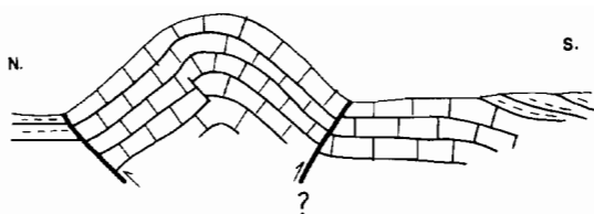
Fig. 2.- Anticlinal de la Sierra de las Cabras.
