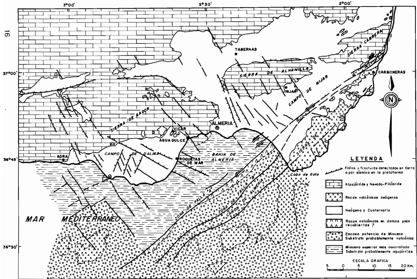
Fig. 1.- Los sistemas de fallos en la costa de Almería durante el Neógeno y Cuaternario (Interpretado según J. Boeno)
