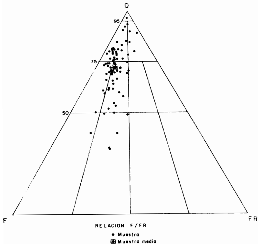
Diagrama de Folk de la Formación T_2^B-Q
