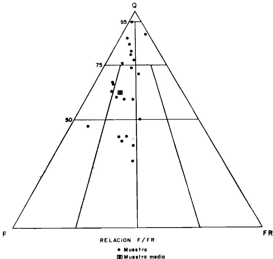
Diagrama de Folk de la Formación Q ca
