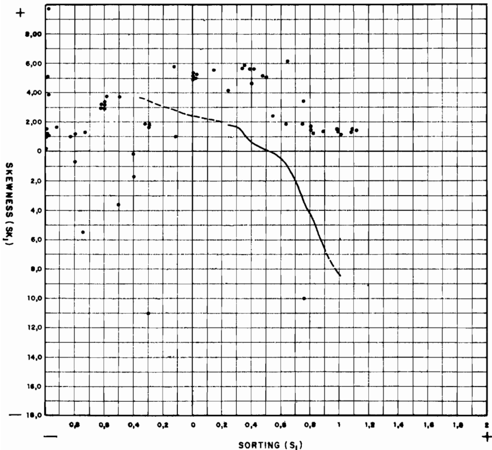
Diagrama Sorting-Skewness de la Formación T_2^B-Q
