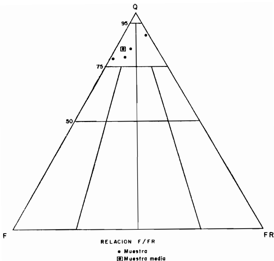
Diagrama de Folk de la Formación T_{12}^{Bc}
