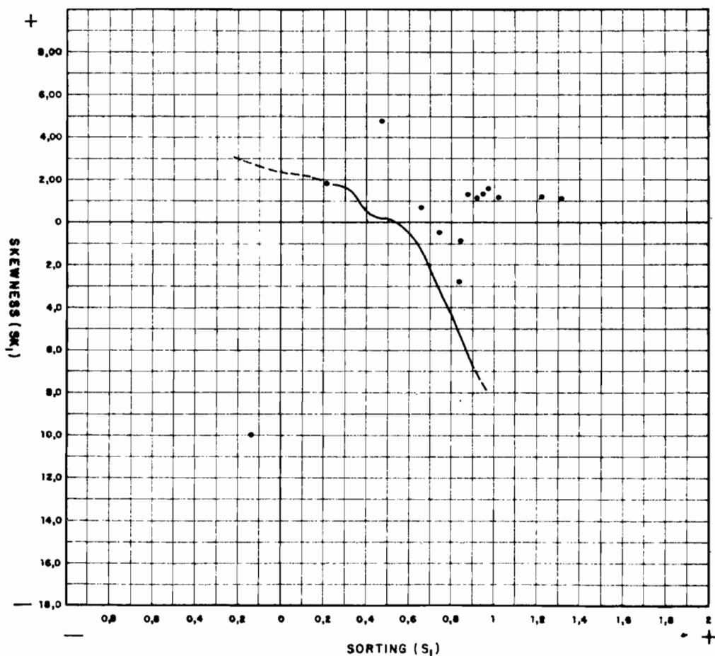
Diagrama Sorting-Skewness de la Formación Qc9
