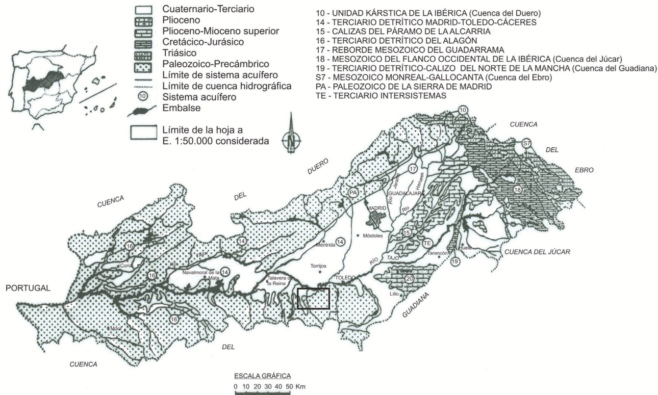
Figura 7.2. - Mapa de situación de los sistemas acuíferos de la Cuenca del Tago de la Hoja de Gálvez.
