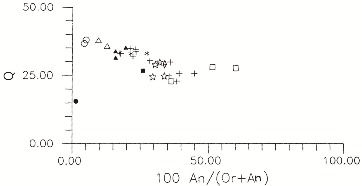
Figura 5.2. - Clasificación de STRECKEISEN y LE MAITRE (1979) a partir de minerales normativos. Simbología: Unidad Migmatítica : Triángulos negros: granodioritas de Layos; Cuadros negros: Granitoides tipo Argés-Guadamur; Círculo negro: cuarzosienita de feldespato alcalino; Rombo: leucogneis. Plutón de Mora-Gálvez: Asteriscos: Granitoides tipo Mora-Menasalbas; Cruces: Granitoides tipo Gálvez; Círculos blancos: Leucogranitos tipo Torcón; Cuadrados: tonalitas; Triángulos blancos: Granitoides tipo San Pablo; Estrellas: Granitoides tipo San Martín. Rombo blanco: Pórfido granítico.
