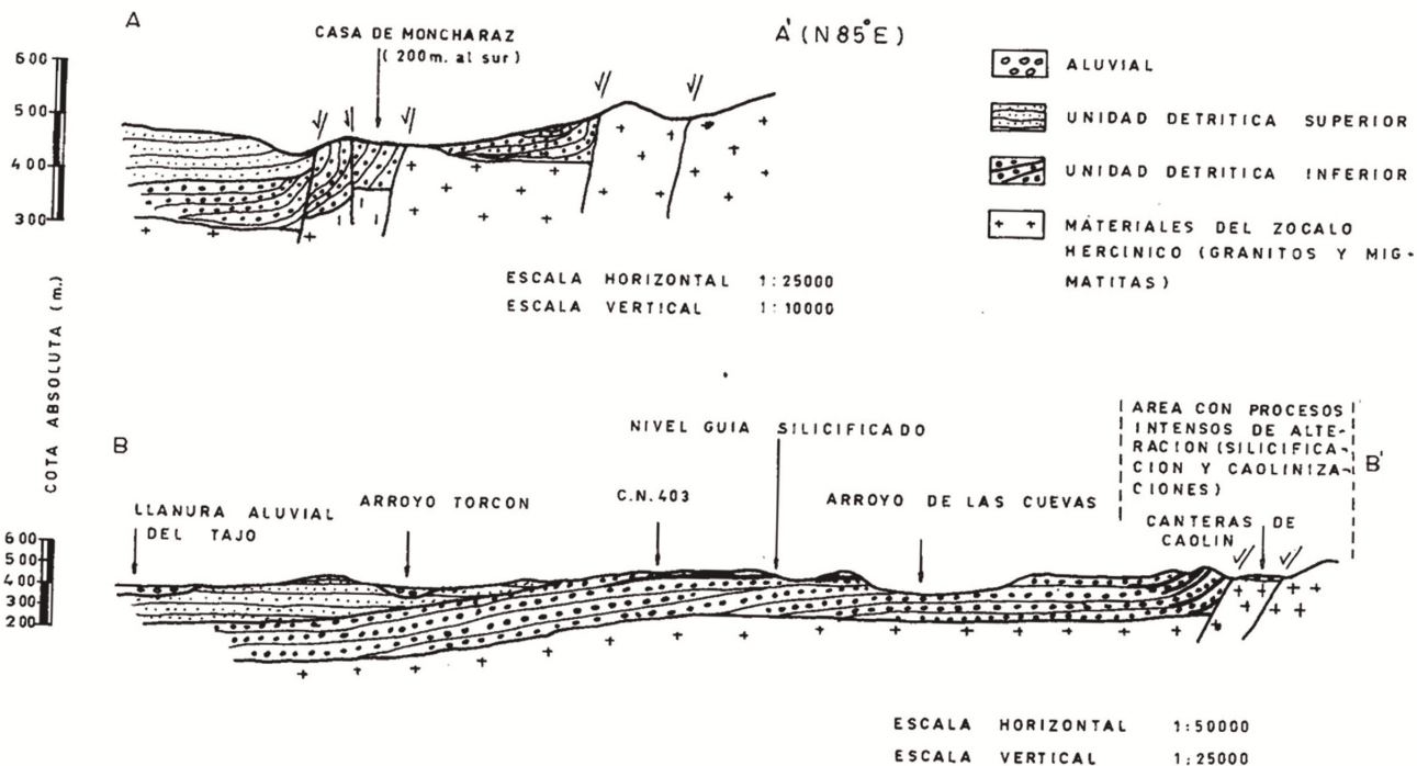
Figura 2.2. - Cortes Geológicos. A) En el contacto en la zona de fracturas "Casa de Moncharaz" Cerro Aguilero. B) Transversal a la cuenca.
