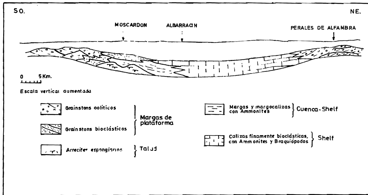
Fig. 3.-Esquema deposicional en el Bajociense superior-Batoniense.
