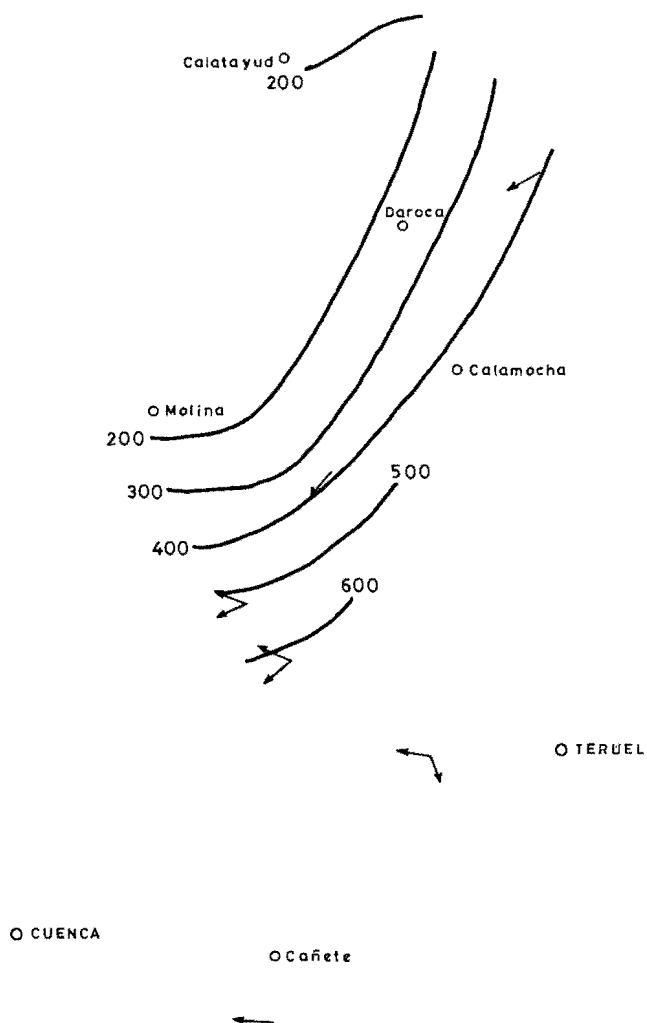
Fig. 5.— Ciclo II. Mapa de isopacas y paleocorrientes.
