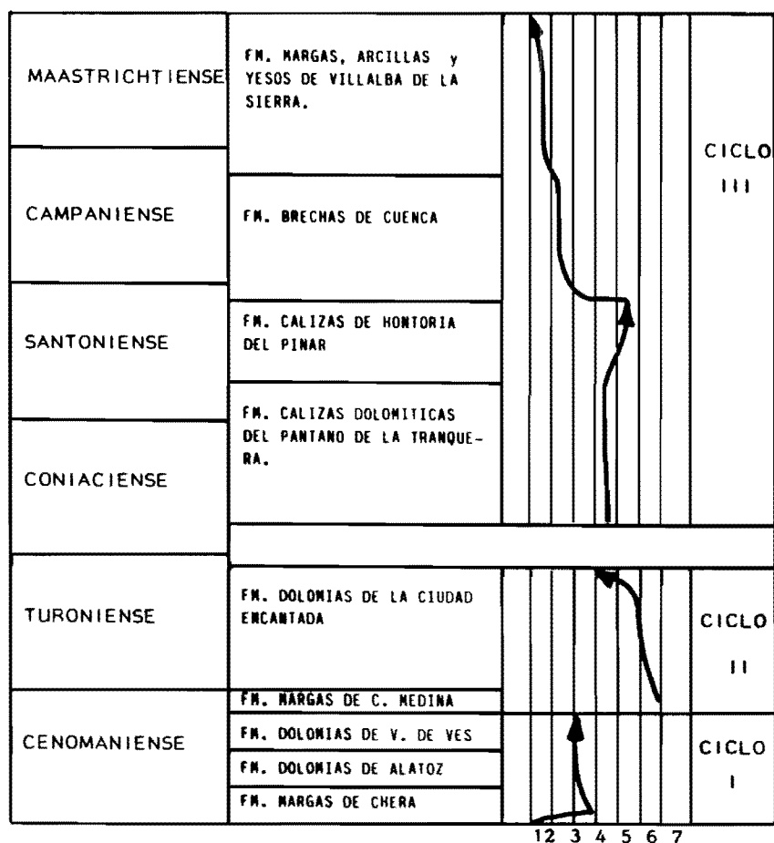
Fig. 5.-Esquema evolutivo de los tres ciclos del Cretácico superior. 1. Continental, 2. Sebkhá, 3. Llanura de mareas, 4. Lagoón, 5. Plataforma interna, 6. Barra, 7. Plataforma externa.
