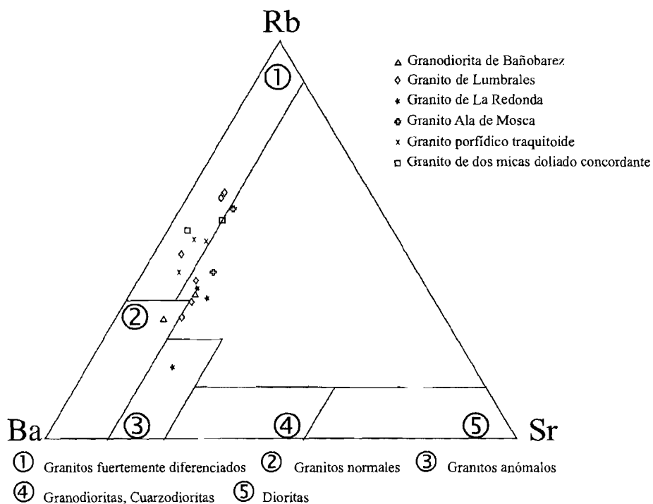
Fig. 2. Diagrama ternario Rb-Ba-Sr (BOUSEILY y SOKKARY, 1975).
