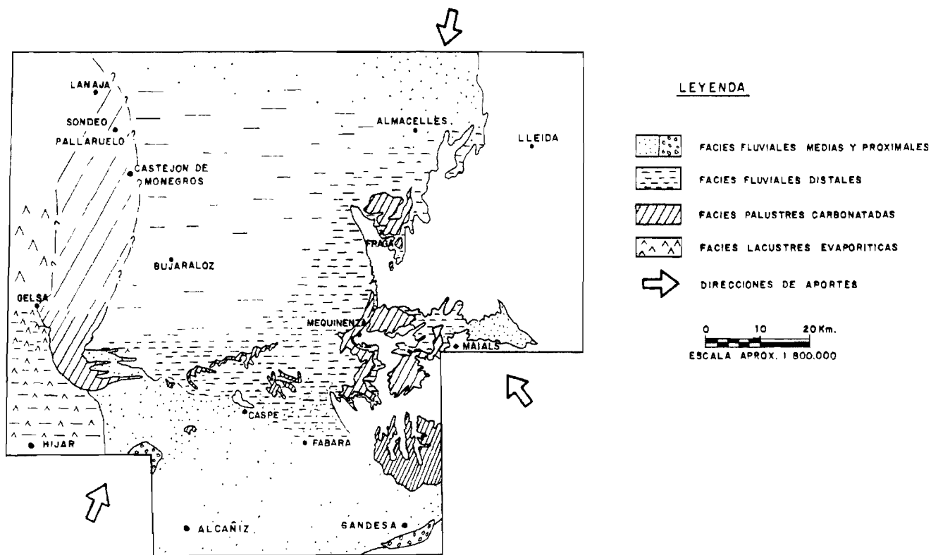
Figura 4. Esquema de distribución de facies de la unidad genético-sedimentaria de Mequinzena-Ballobar.
