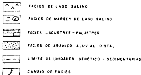
Figura 2. Modelo secuencial de las unidades genético-sedimentarias del sector sur de Los Monegos.
