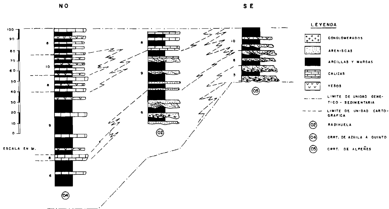
Figura 8. Evolución lateral y vertical de la unidad genético-sedimentaria de Torrente de Cinca-Alcolea de Cinca en la hoja de Híjar
