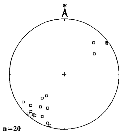
Fig. 14. Proyección estereográfica equiareal de elementos estructurales de D1 (L1) medidos en materiales de la Unidad Inferior. a) Ermita de Pereña, b) Cerro Tabanera.
