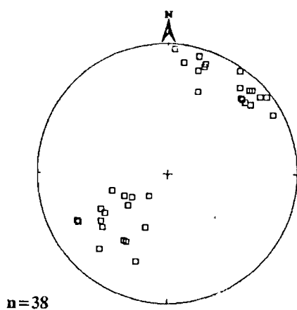
Fig. 14. Proyección estereográfica equiareal de elementos estructurales de D1 (L1) medidos en materiales de la Unidad Inferior. a) Ermita de Pereña, b) Cerro Tabanera.
