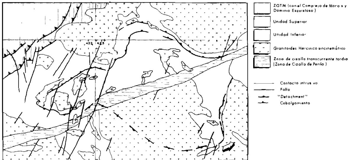
Fig. 1 Mapa estructural esquemático del Domo Gneisico del Torres (modificado de ESCUDER, 1995)
