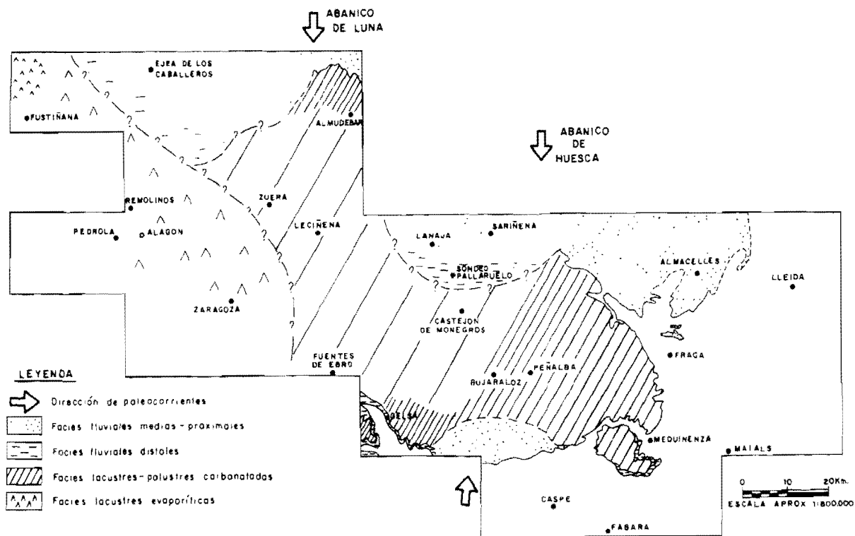
Fig. 8. Esquema regional de distribución de facies de la unidad genético-sedimentaria de Torrente de Cinca-Alcolea de Cinca
