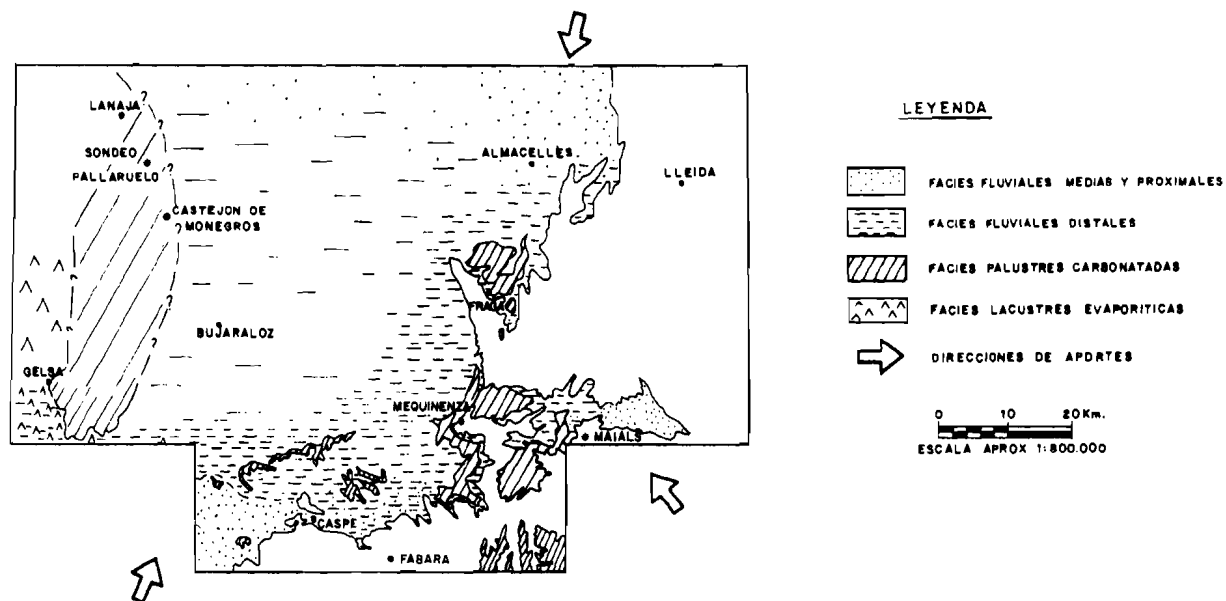
Fig. 7. Esquema regional de distribución de facies de la unidad genético-sedimentaria de Mequinenza-Ballobar
