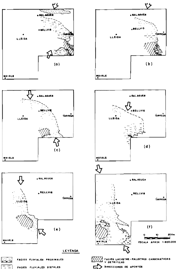
Fig. 5. Esquemas de distribución de facies de las unidades genético-sedimentarias de Vallbona (a), Omells (b), Floresta (c), Arbeka (d), Castellans (e) y Alfés (f)
