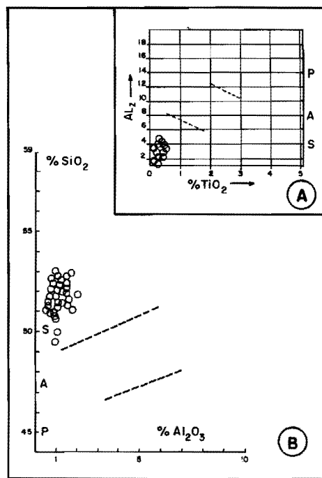
Fig.-13 Expresión de la composición de los ortopiroxenos: A) Relación alúmina-titanio (diagrama de Le Bas, 1962) para los piroxenos de la fig. 9 B) Relación sílice-alúmina para los mismos piroxenos (diagrama de Nisbert y Pearce, 1977); S = dominio subalcalino. A = alcalino y P = paralcalino.
