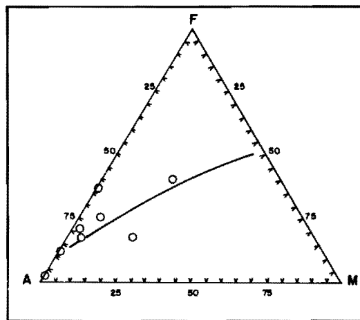
Fig.- 17 Diagrama AFM mostrando la afinidad calcoalcalina de estas rocas
