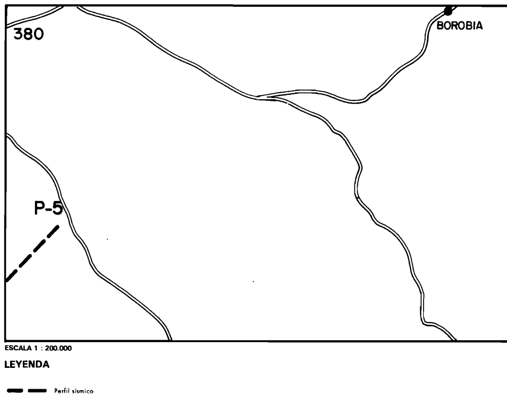
Fig.-1 Esquema de situación de los perfiles sísmicos en la Hoja de Borobia (380)
