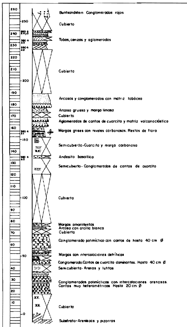
Fig.- 3 Serie volcánoclastica en el arroyo Ruidero (según LAGO y POCOVÍ)
