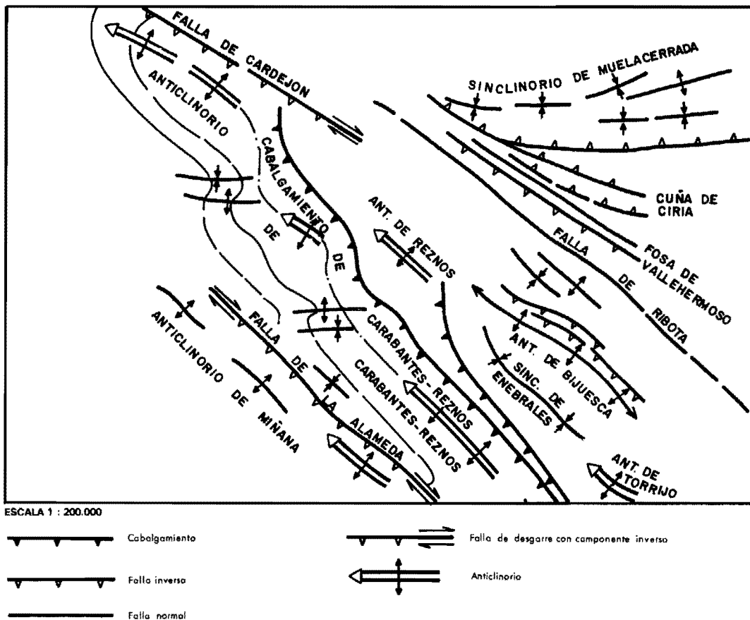
Fig.- 10 Principales estructuras
