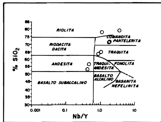
Fig.-15 Clasificación de las rocas según la relación SiO_2 -Nb/Y
