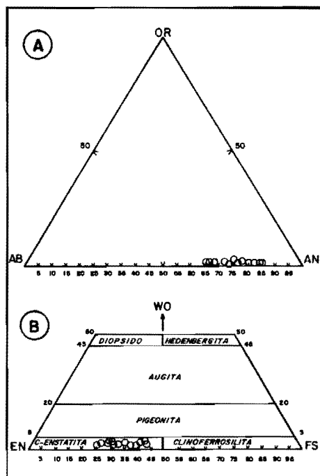
Fig.- 12 Análisis de microsonda en A) Plagioclasas, B) Ortopiroxenos. Dique de andesita basáltica del Arroyo del Ruidero.
