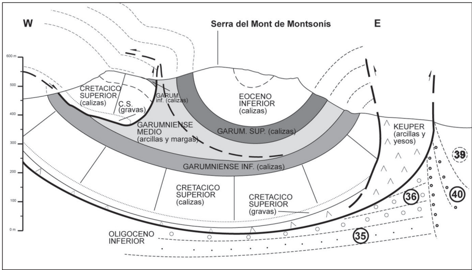
Fig. 2.- Corte geológico de la Lámina de Montsonis-Serra Mosquera. Los números en círculos se refieren a las unidades cartográficas descritas en la memoria.
