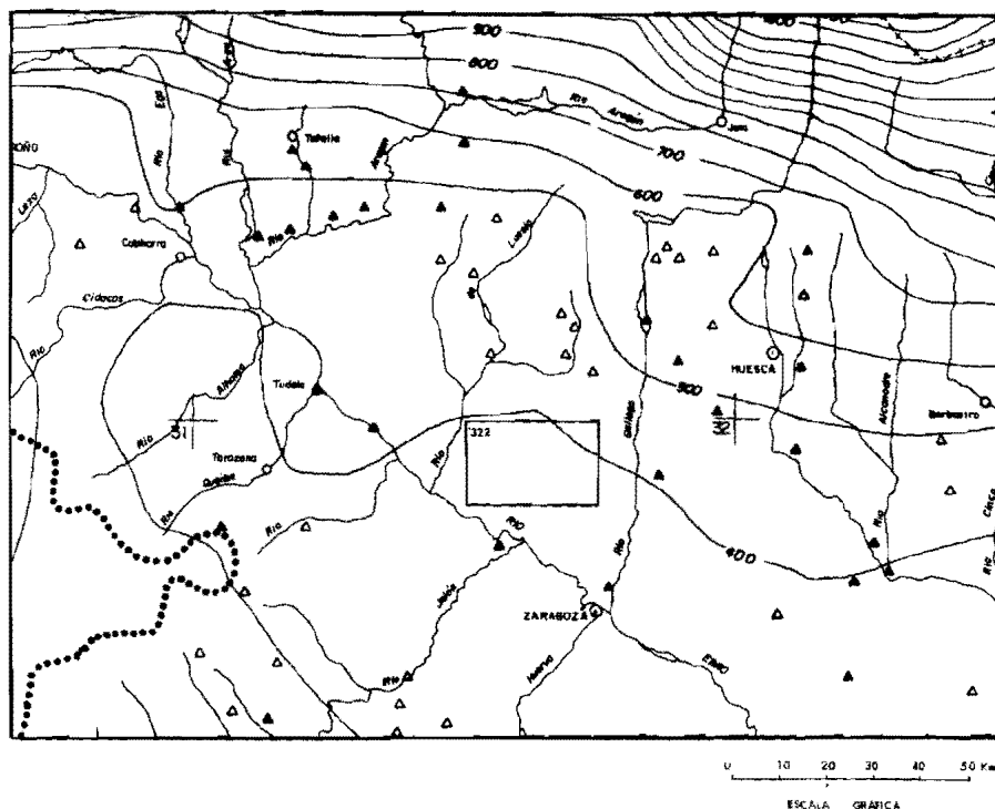
Mapa regional de isoyetas medias
