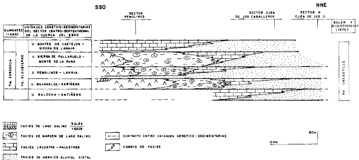
Fig. 2. Modelo secuencial de las unidades genético-sedimentarias miocenas en el sector noroccidental de la parte aragonesa de la cuenca del Ebro
