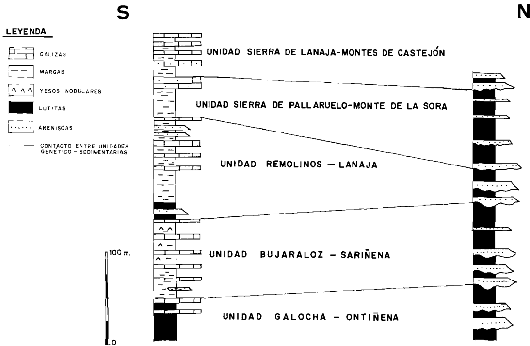
Fig. 4. Columnas sintéticas de las unidades genético-sedimentarias en los sectores septentrional y meridional de la hoja de Ejea de los Caballeros
