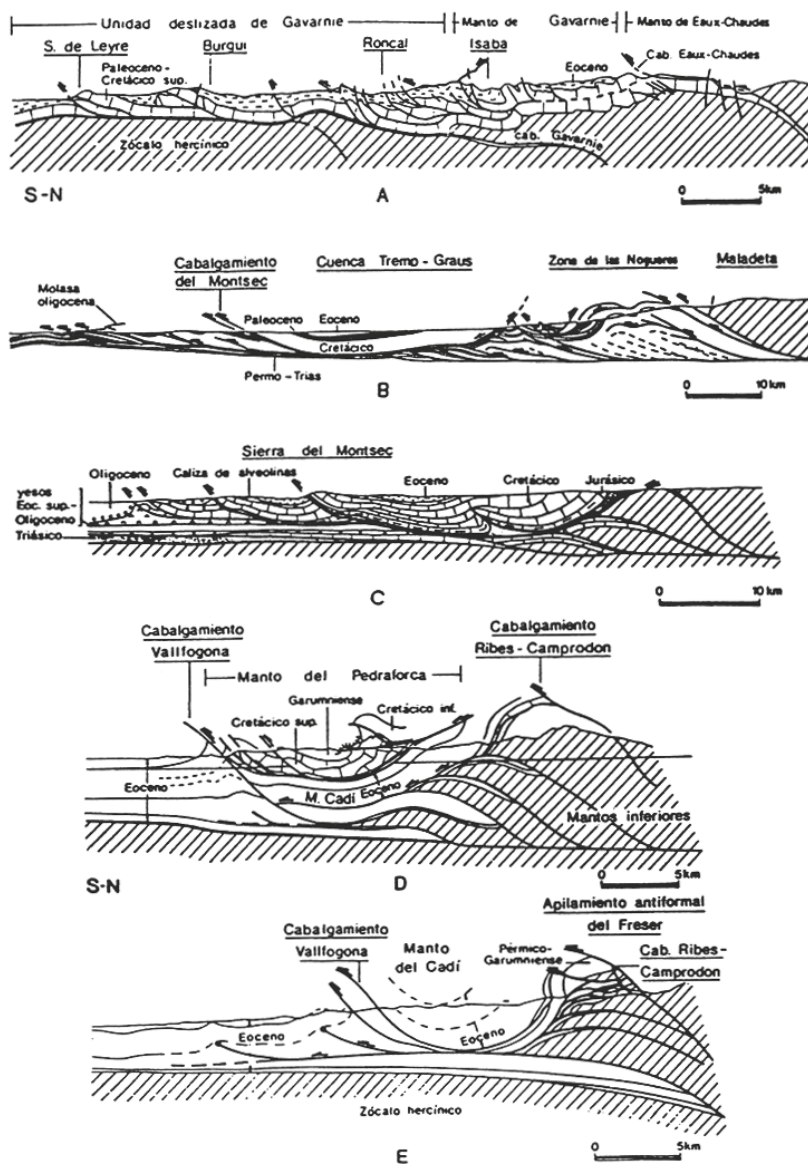
Fig. 10.- Cortes geológicos de la vertiente surpirenaica del Pirineo central (A, B y C) y del Pirineo oriental (D y E). A. LUBAUME y SEGURET (1985), simplificados; B. WILLIAMS (1985), C. CÁMARA y KLIMOWITZ (1985), D. VERGES y MARTÍNEZ, en prensa (Figura procedente de MUÑOZ et al., 1983).
