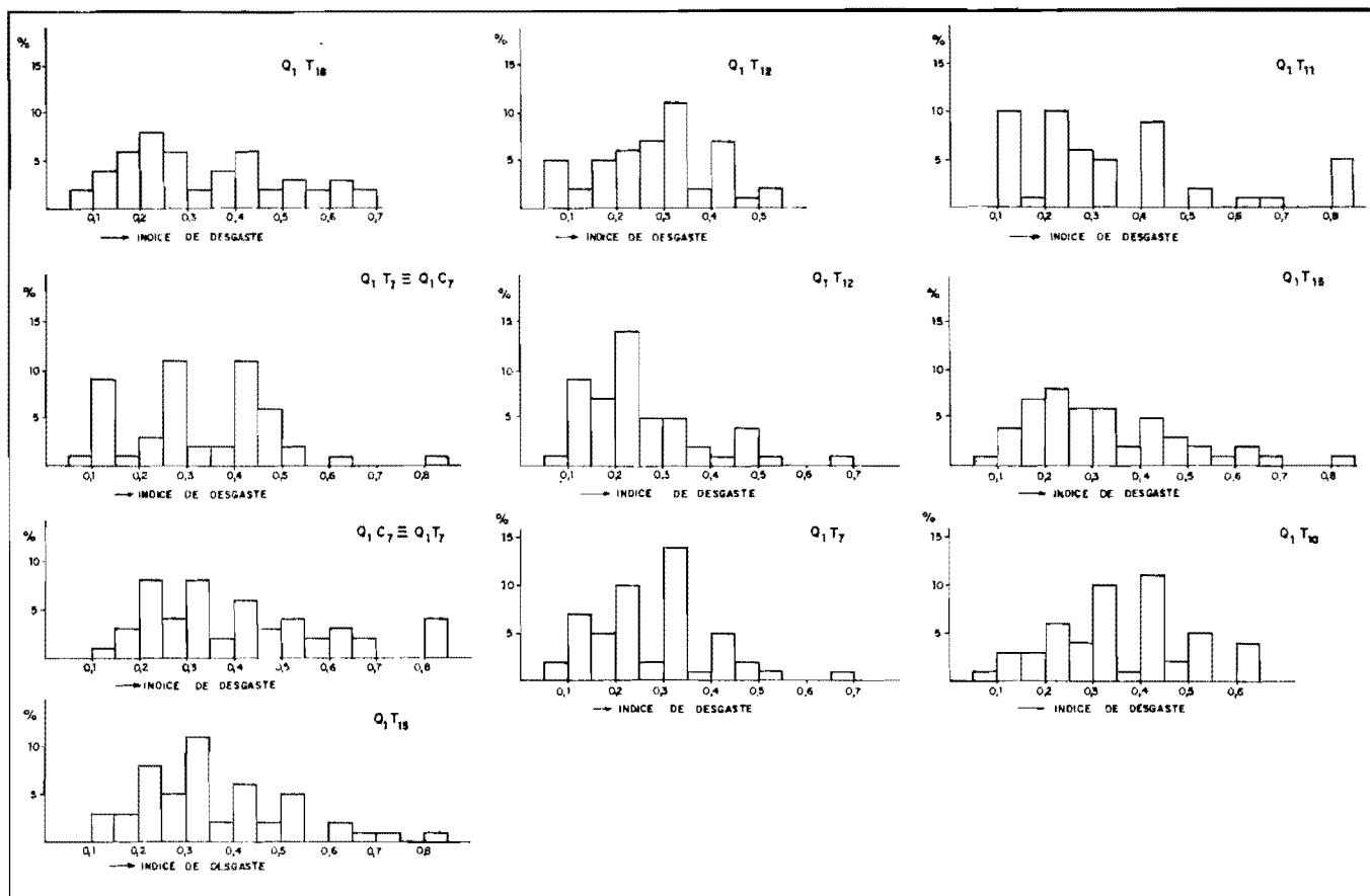
Figura 8.—Histogramas de índices de desgaste. (Hojas 16-11, 16-12 y 16-13).
