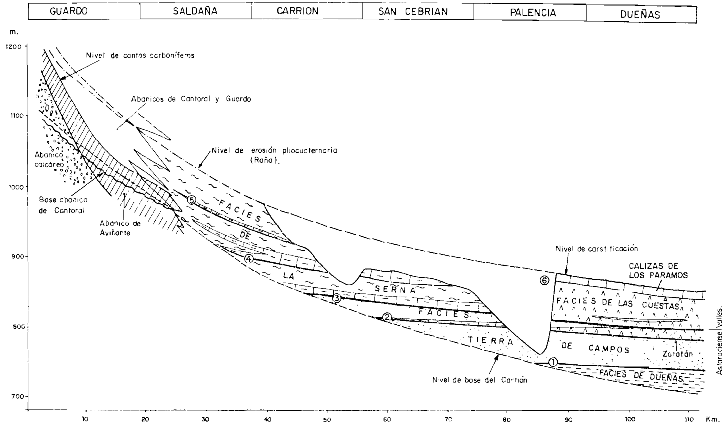
Figura 1.—Esquema estratigráfico.
