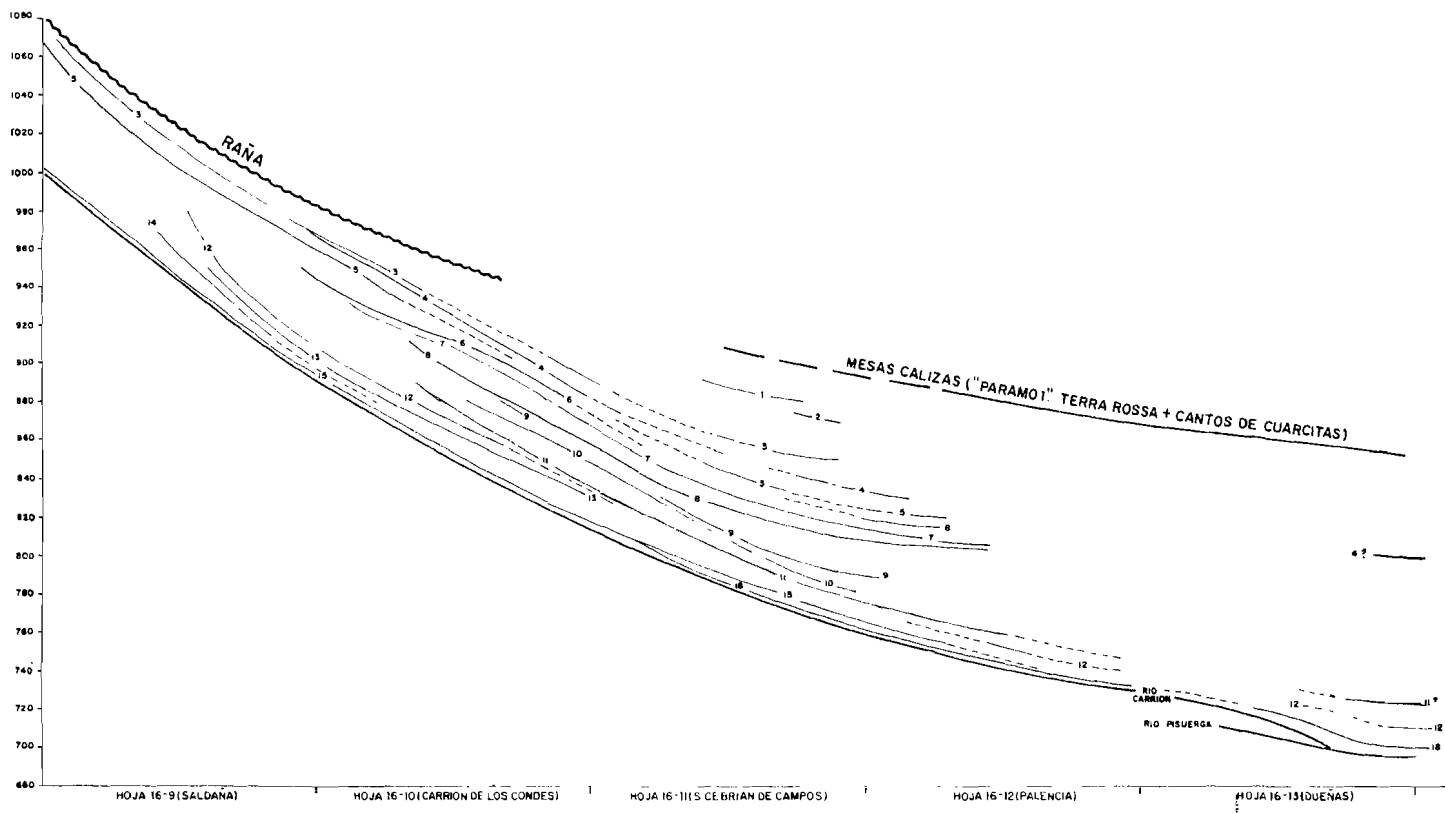
Figura 7.—Perfil longitudinal de las principales terrazas del río Carrilón.
