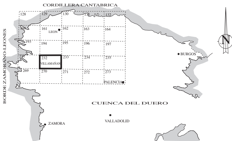
Fig. 1.- Situación de la Hoja N° 232 (Villamañán) en el ámbito de la Cuenca del Duero.
