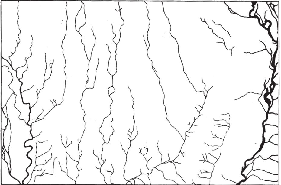
Fig. 10.- Esquema de la red de drenaje de la Hoja de Villamañán.
