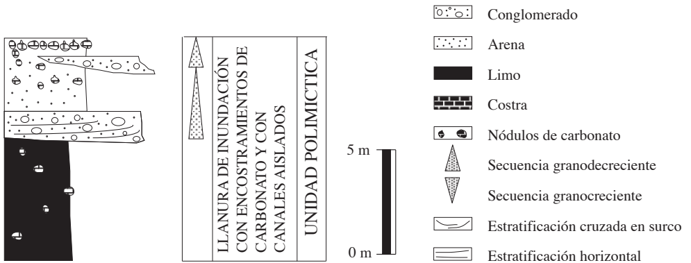
Fig. 5.- Columna estratigráfica de la Unidad Polimíctica (1) en la localidad de Castrofuerte.
