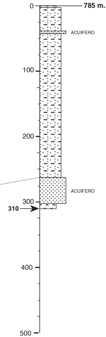
Fig. 14.- Propuesta de correlación entre los distintos acuíferos del subsuelo de la Hoja de Villamañán. Según Redondo et al. (1995).
