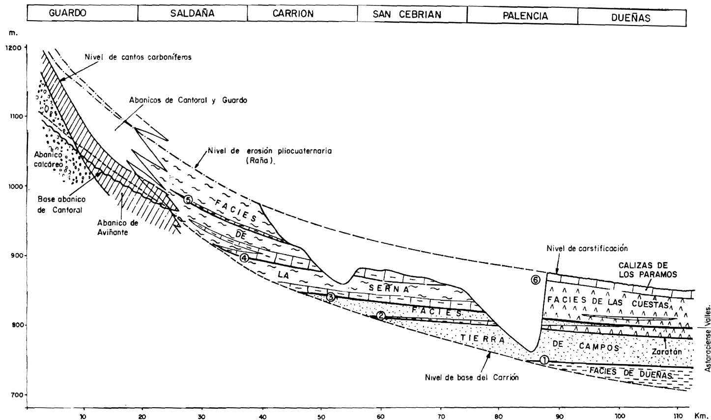
Figura 10.—Esquema estratigráfico. Núms. 1 a 6. Líneas aproximadamente isócronas. Núm. 3. Base del Vallesiense.
