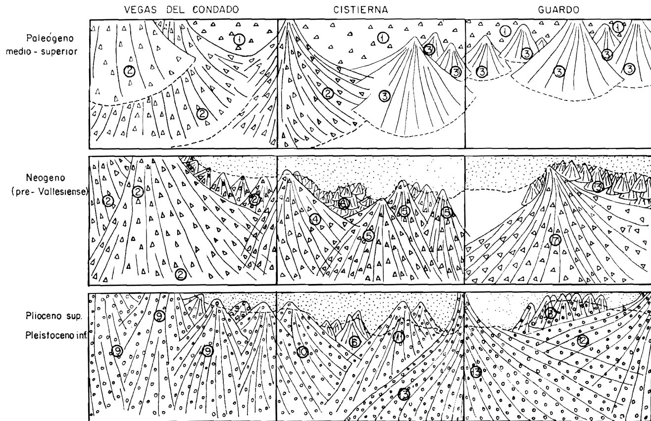
Figura 8.—Esquema paleogeográfico.
