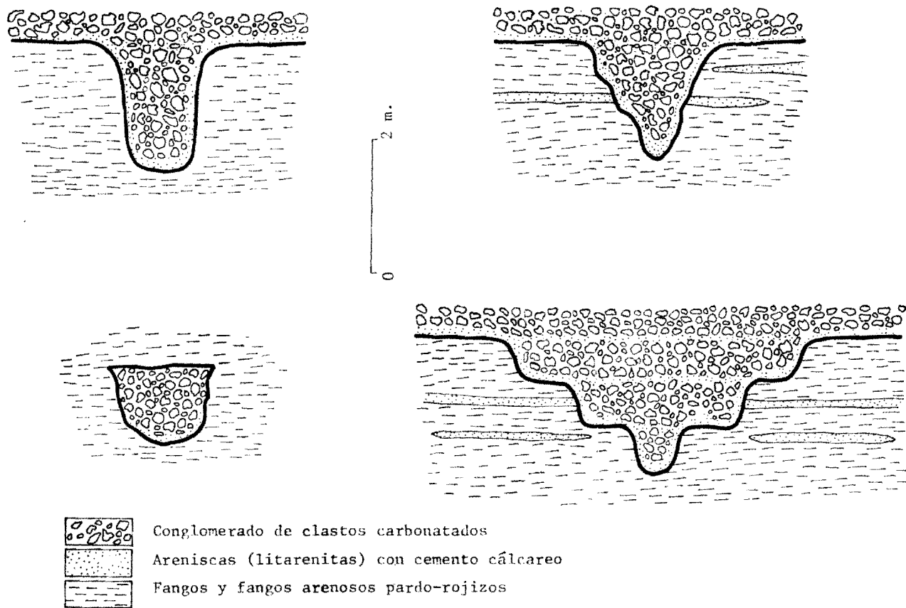
Figura 1.—Secciones más comunes, transversales, de canales en las áreas intermedias de los abanicos del Complejo de Cuevas y de Avilante.
