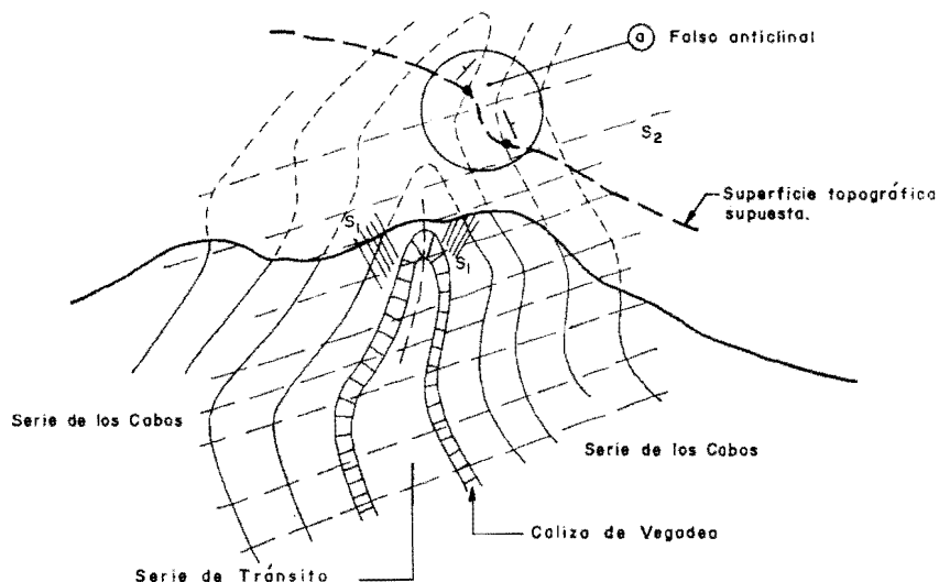
Figura 4.—Anticlinal de Fase 1 con flexiones causadas por la S_2 , que ha basculado la S_1 , en la zona de Ancares.
