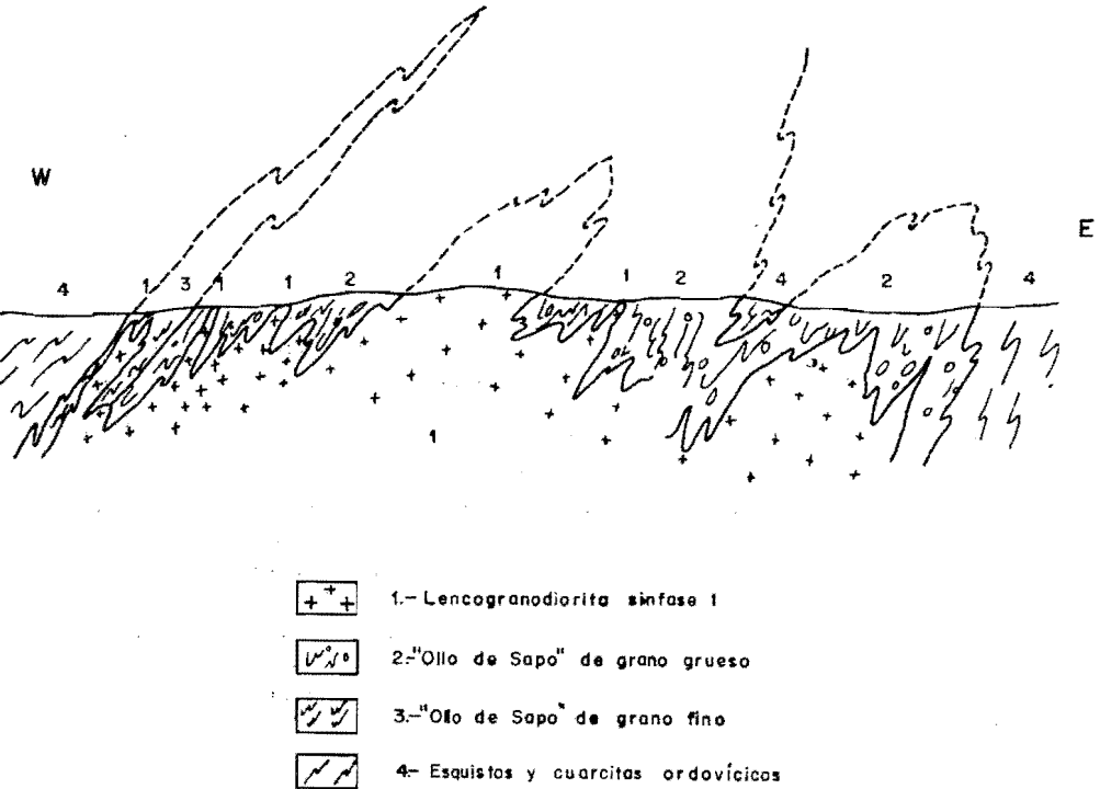
Fig. 4.—Corte esquemático de la zona axial del anticlinal del «Ollo de Sapo».
