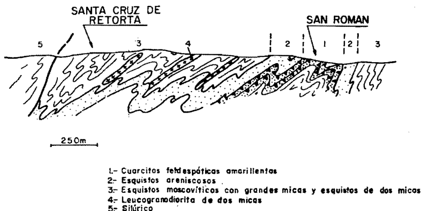
Fig. 2.—Corte esquemático de la «Serie de Alba», por Retorta.
