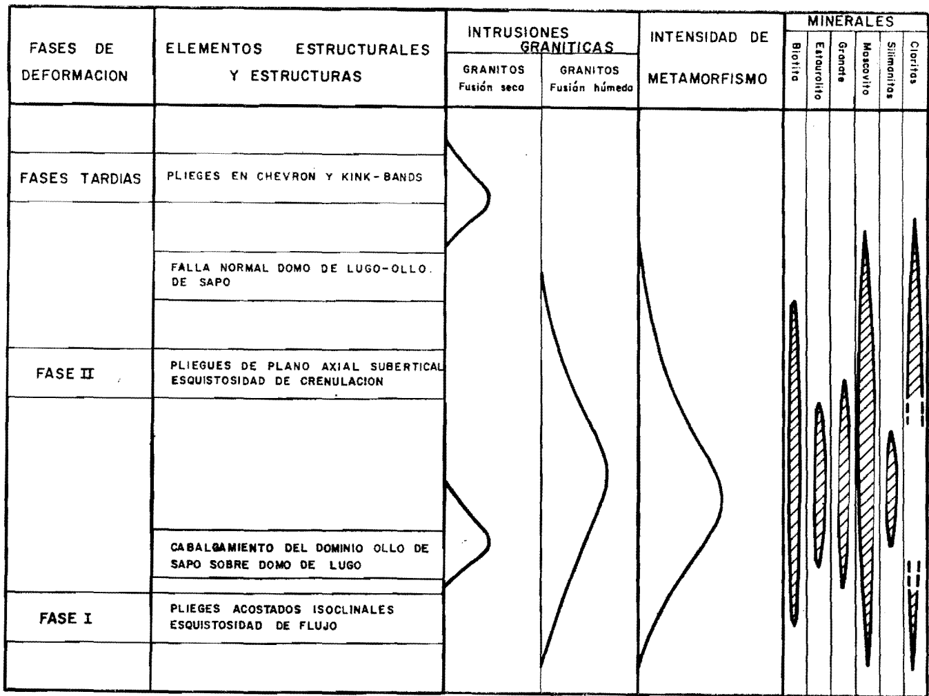
Fig. 9.—Relaciones entre las fases de deformación, emplazamiento de granitos, intensidad de metamorfismo y aparición de minerales de metamorfismo.
