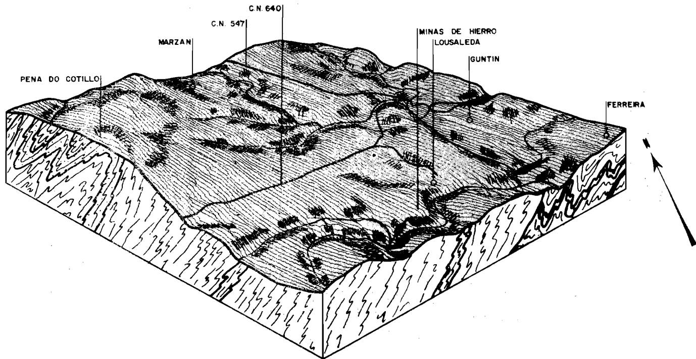
Fig. 8.—Bloque diagrama del sector de Guntin, en la parte central de la Hoja. Dominio del «Olló de Sapo».
