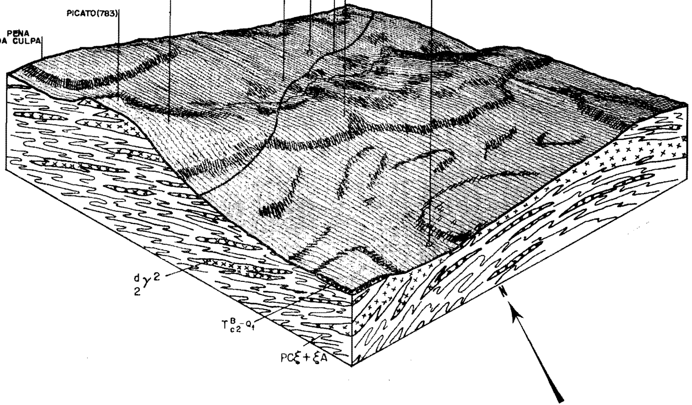
Fig. 7.—Bloque diagrama del sector Calde Castelo, en la parte central de la Hoja. Dominio del «Domo de Lugo».
