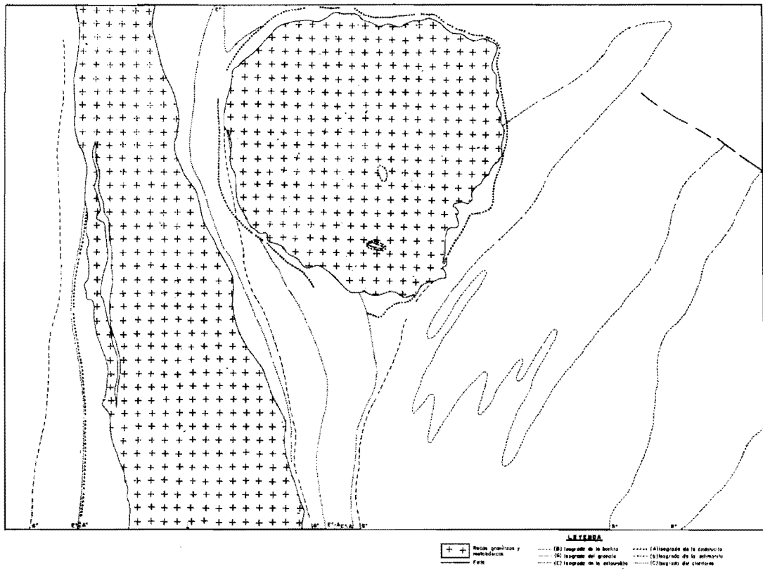
Fig. 1.—Desarrollo de las isogradas de la Hoja de Puente deume.
