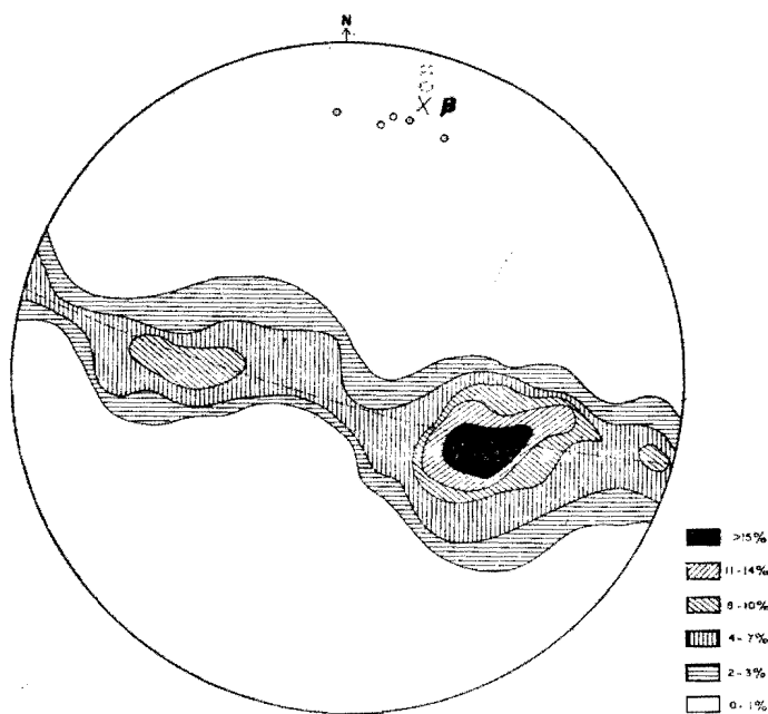
Fig. 5.—Diagrama de polos a planos S_0 en la serie de Ordenes en las proximidades de playa Almeiras con cinco ejes de pliegues (o) B_1^2 (55 polos).
