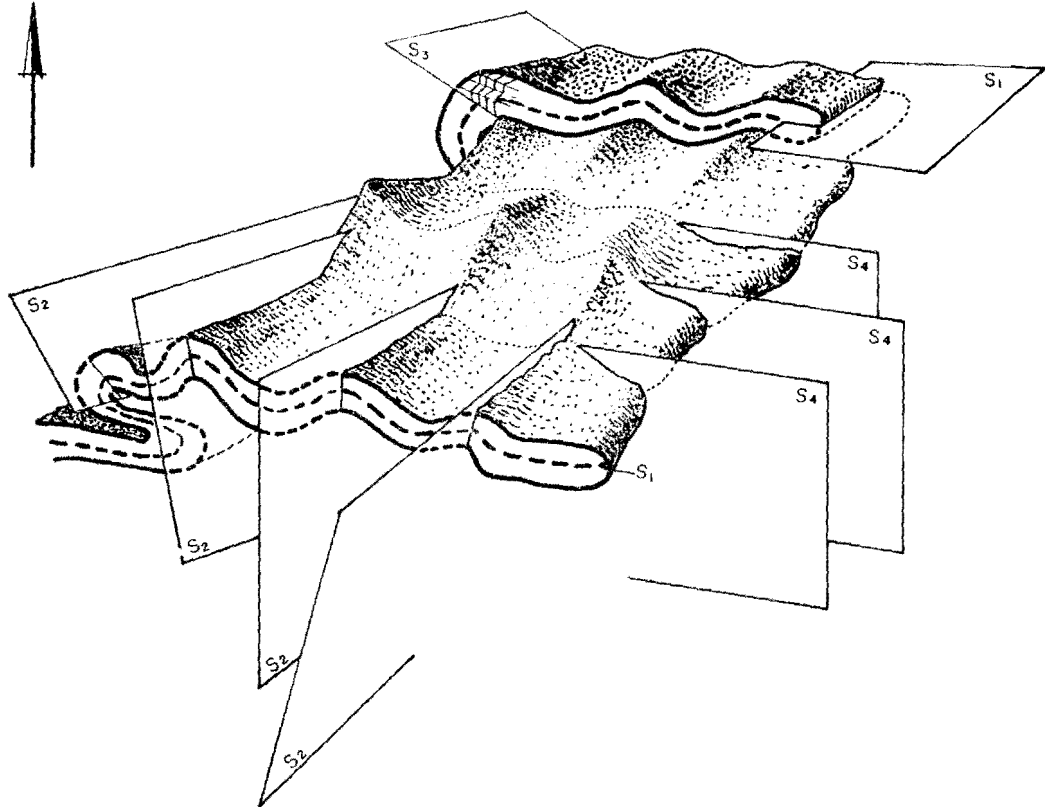
Fig. 2.—Esquema de la superposición de las cuatro fases de deformación en la Hoja de Puente deume.
