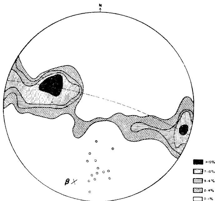
Fig. 4.—Distribución de S_0 (estratificación) en los materiales cuarcíticos del Ordovícico Inferior ( O_{12}^2\gamma ), al este de Taboada con 14 ejes B_1^2(0) (58 polos).
