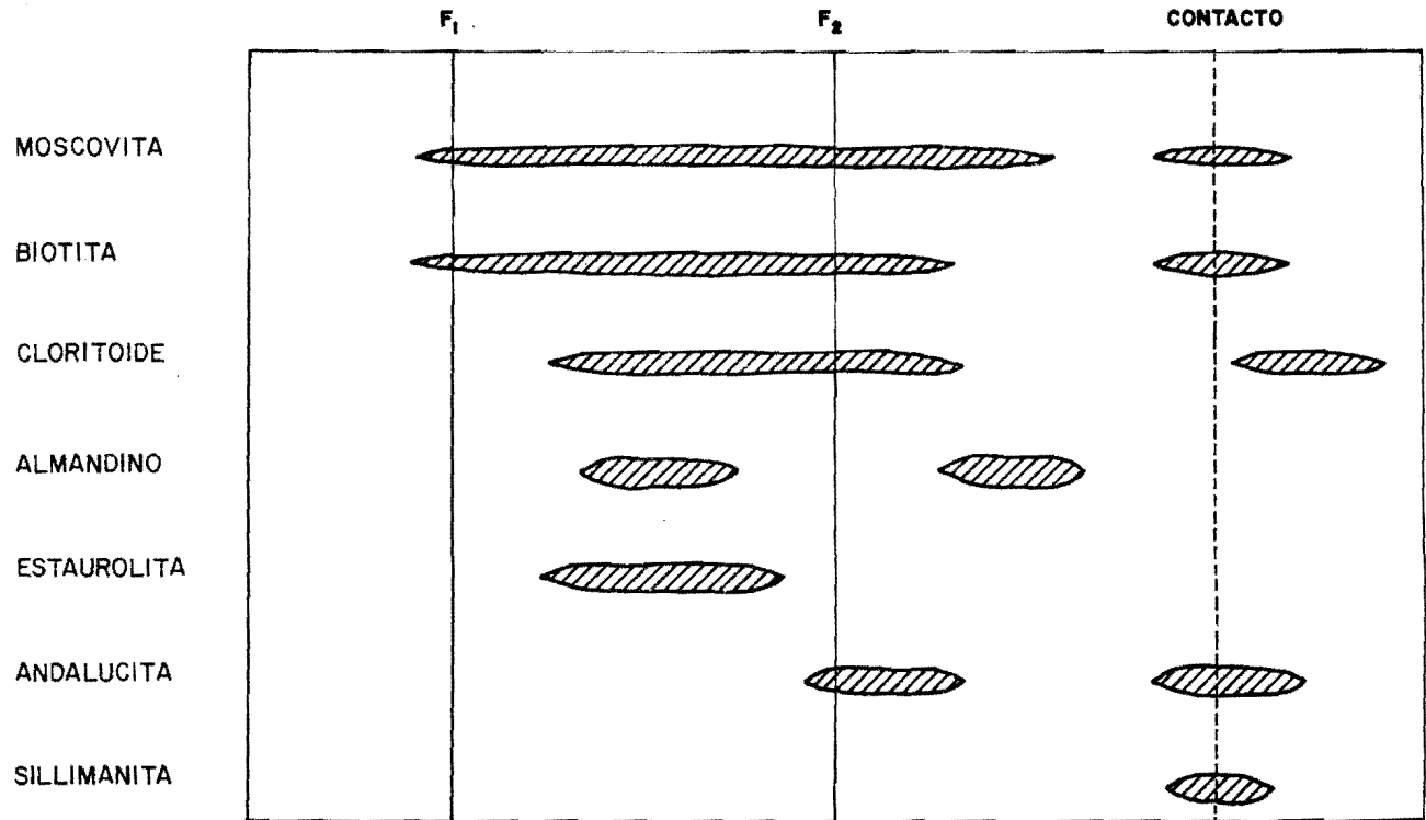
Fig. 8.—Esquema de crecimiento de minerales respecto a las deformaciones.
