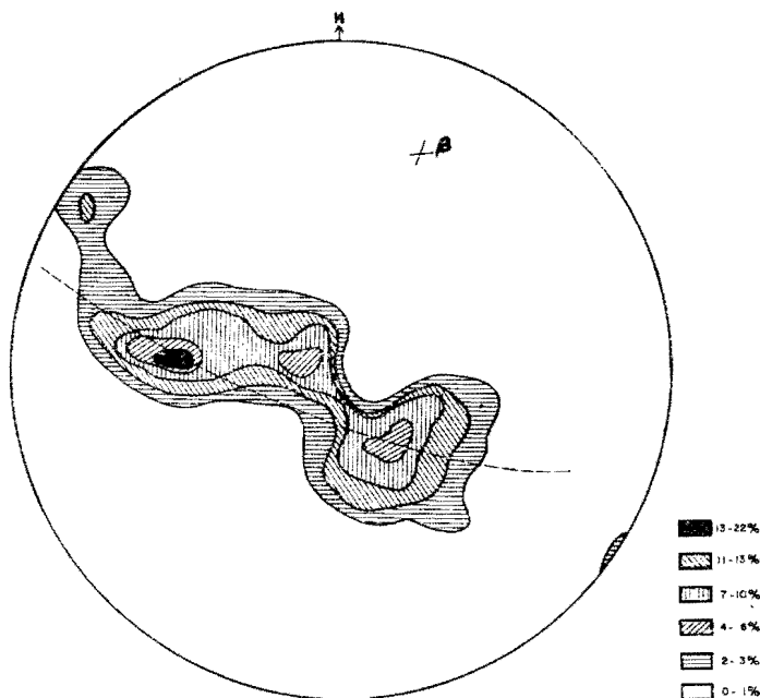
Fig. 3.—Diagrama de polos a planos S_0 (estratificación), entre Reboredos y Ferreiros (71 polos). Diagrama 1.
