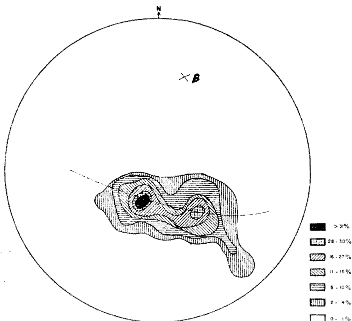
Fig. 7.—Diagrama de polos a planos S_1 (esquistosidad primaria) en el Silúrico, entre San Pedro y Piedramayor (84 polos). Diagrama 3.
