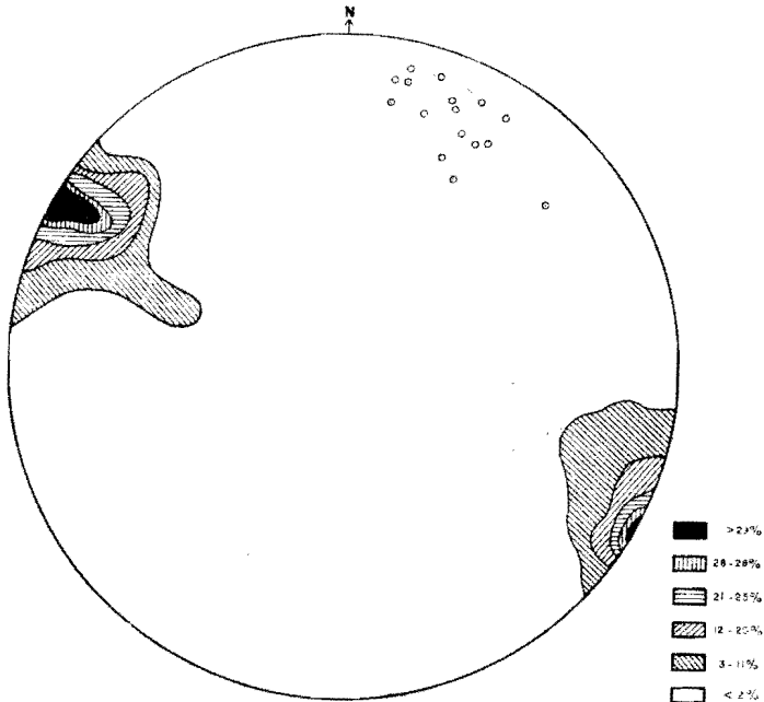
Fig. 6.—Diagrama de polos a planos S_2 (esquistosidad secundaria) con 16 ejes de pliegue (o) B_1^2 , entre Rebaredos y Ferreiros (34 polos). Diagrama 2.
