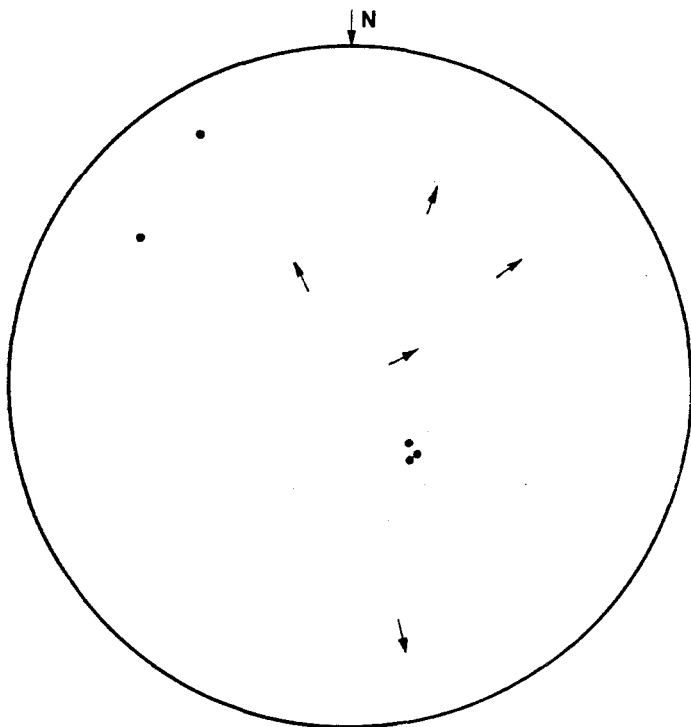
Diagrama 11.— \cdot = S_3 \rightarrow = L_2
