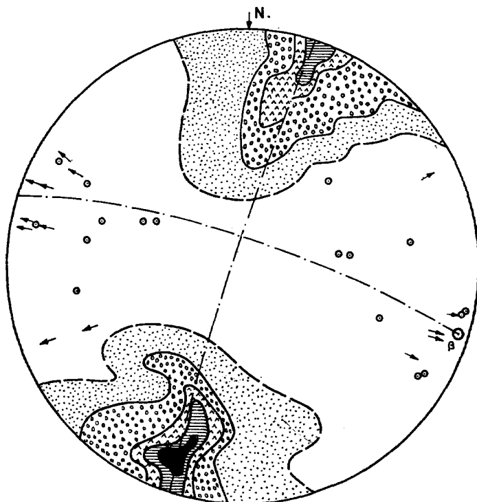
Diagrama 4.—54 polos de S_1 (contornos 0, 1, 2, ... 4%), 14 L_1 (→) y 17 L_3 (○) en el Infracámbrico noroccidental.
