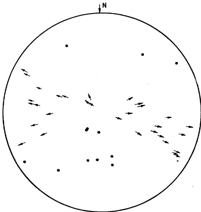
Diagrama 10.— \bullet = S_4 \rightarrow = L_3
