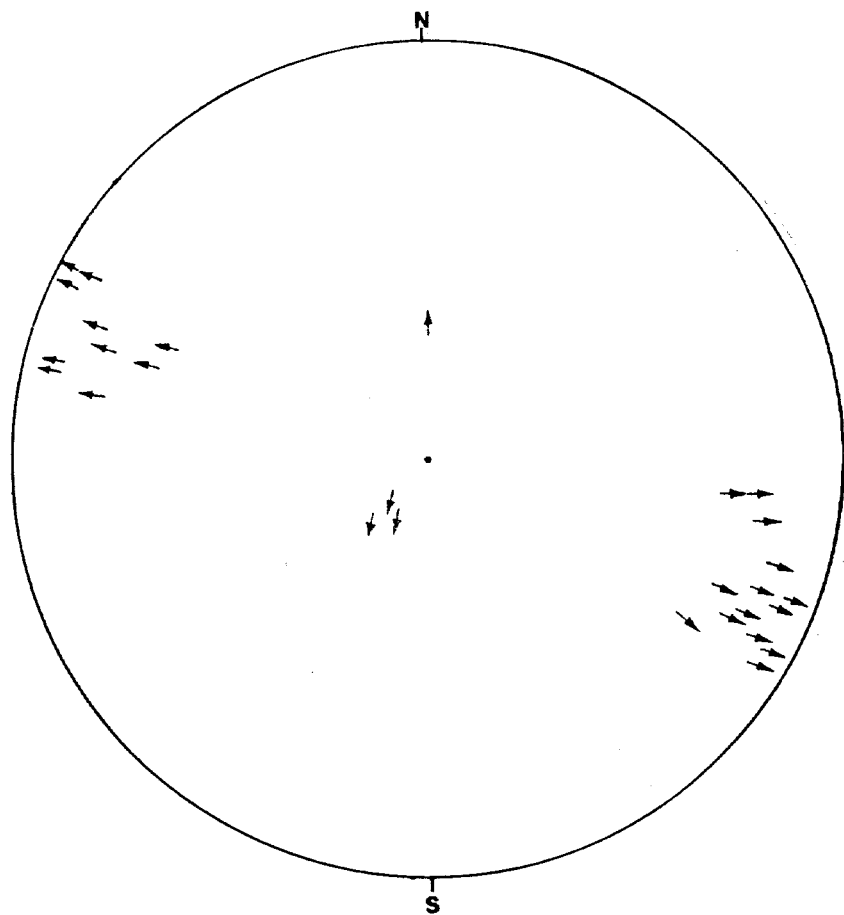
Fig. 3.—Proyección sobre el hemisferio inferior de la red de Schmidt de 24 ejes B_3 (3. a fase) y cuatro ejes B_2 (2. a fase).
