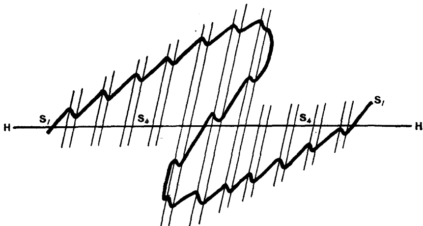
Fig. 4.—Pliegues mesoscópicos asimétricos de plano axial S_4 (3.ª fase) superpuestos a pliegues macroscópicos (1.ª fase). (Adaptado de TURNER, F. y WEIS, L., 1963, fig. 5-32, p. 191.)
