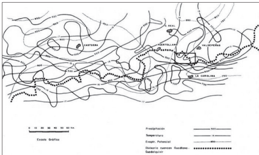
Fig. 7.1.- Mapa regional de isoyetas, isotermas y E.T.P.
