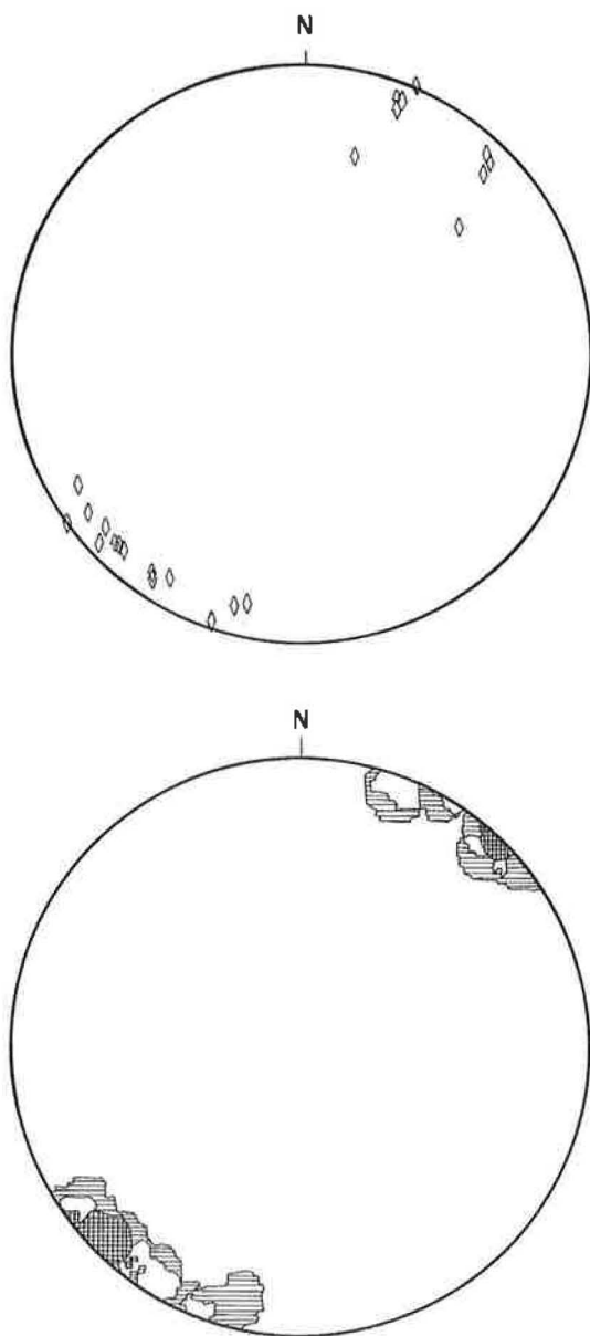
Fig. 3.7. Representación estereográfica de 28 polos de S_1 en las Unidades de Arroyo Fresneda y Sierra Bermeja. Proyección del hemisferio inferior. Contornos del 4, 11 y 18%.
