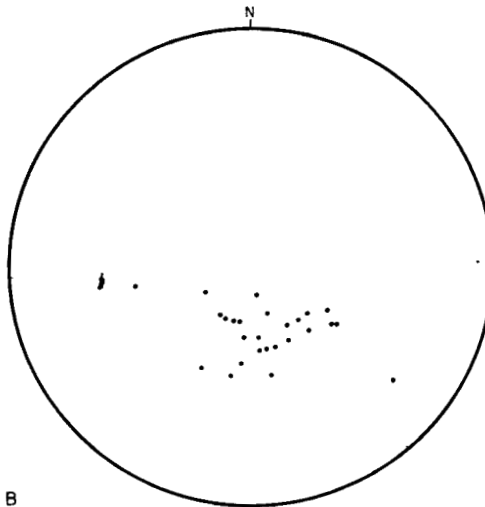
Figura N° 6 A.- Proyección equiareal de los polos (22) de la foliación y bandeo de las migmatitas y anatexitas de Azutan. B.- Proyección equiareal de los polos (26) de la fluidalidad planar del granito de Aldeanueva de Barbarroja.
