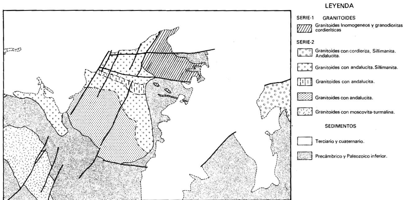
FIGURA N° 8. Distribución de las fases aluminicas. (Modificado de ANDONAEGUI-BARRERA 1984).
