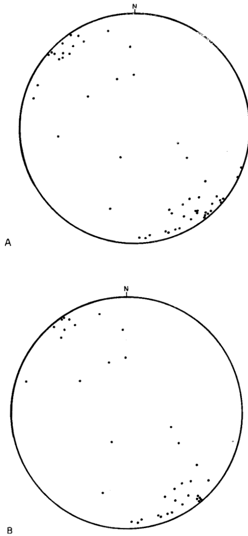
FIGURA N° 4.- Proyección equiareal de la lineación L (58) en la Formación Limolitas del Pusa (Arroyo de Fuentes, Río Huso y corte del F.C.) B.-Lineación L (39 Polos) en los Fm. Limolitas del Pusa (Arroyo de Fuentes, Río Huso y corte de F.C.)
