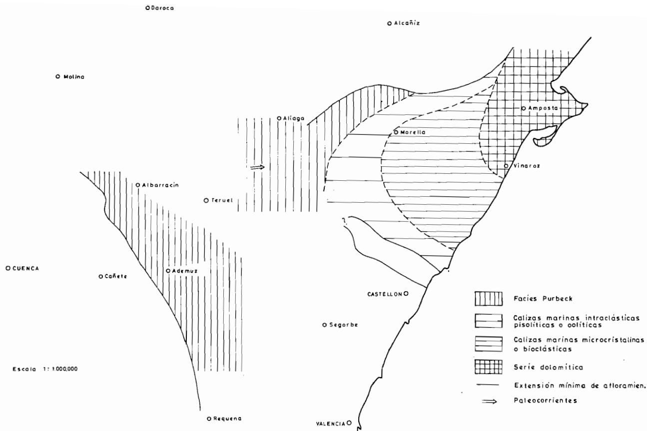
Fig. 8.— Mapa de facies y extensión mínima de los terrenos del Portlandiense-Cretácico basal. Datos de VIALLARD, CANEROT y propios.
