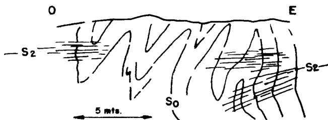
Figura 2.—Pliegues de fase I deformados por la fase II. Carretera de Presa das Portas.
