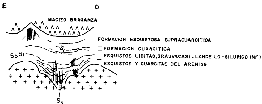
Figura 3.—Esquema de situación del Sinclinorio de Verin al fin de la fase III.
