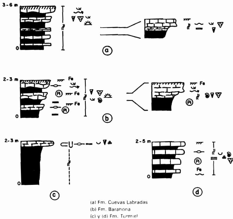
Figura 1. Secuencias tipo de la unidad cartográfica núm. 15.
