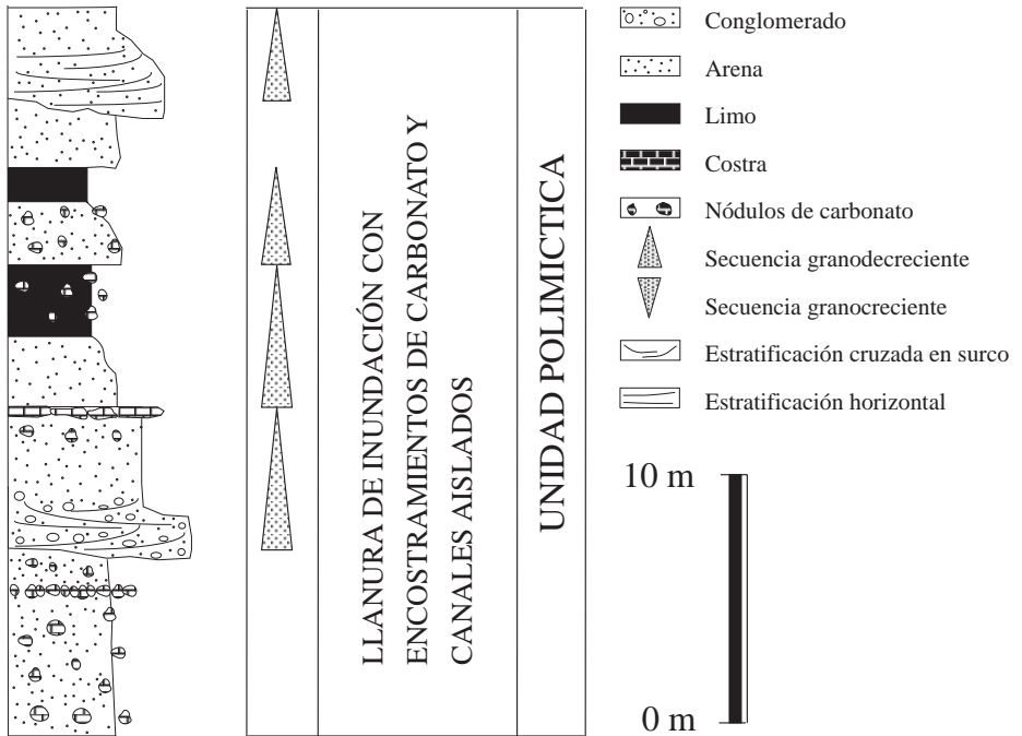
Fig. 3.- Columna estratigráfica de la Unidad Polimíctica (1) en la localidad de Villalobar.
